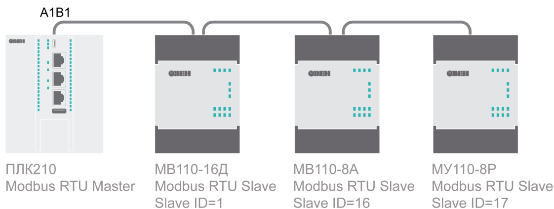
Рисунок 6.1 – Структурная схема примера
