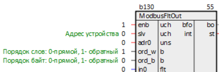
Рисунок 3.18 – Блок ModbusFltOut
