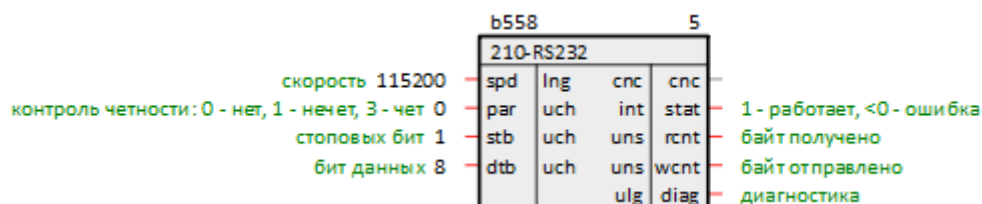
Рисунок 2.2 – Порт RS-232 (210-RS232)
