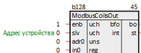
Рисунок 3.16 – Блок ModbusCoilsOut
