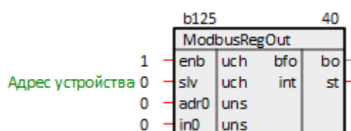
Рисунок 3.15 – Блок ModbusRegOut
