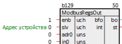
Рисунок 3.17 – Блок ModbusRegsOut
