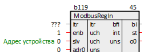
Рисунок 3.10 – Блок ModbusRegIn
