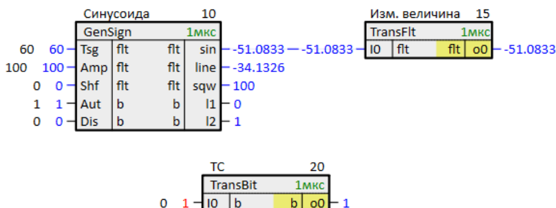
Рисунок 3.25 – Успешный обмен данными. Сервер
