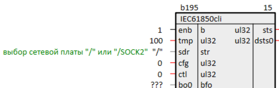
Рисунок 2.11 – Блок IEC61850cli
