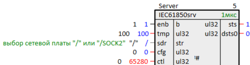
Рисунок 5.1 – Включение вывода всех диагностических сообщений сервера
