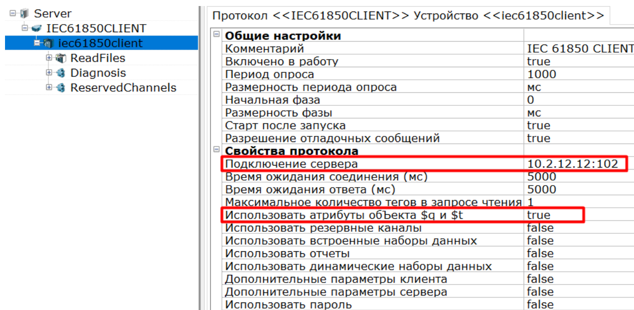
Рисунок 3.39 – Настройка iec61850client
