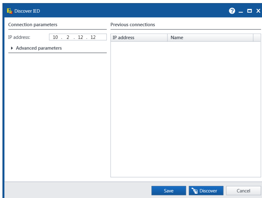
Рисунок 3.21 – Поиск устройства 61850
