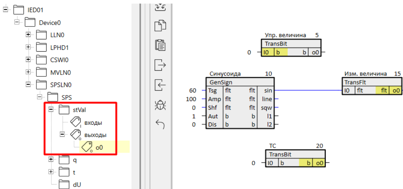
Рисунок 3.13 – Связь атрибута данных класса SPS с TransBit
