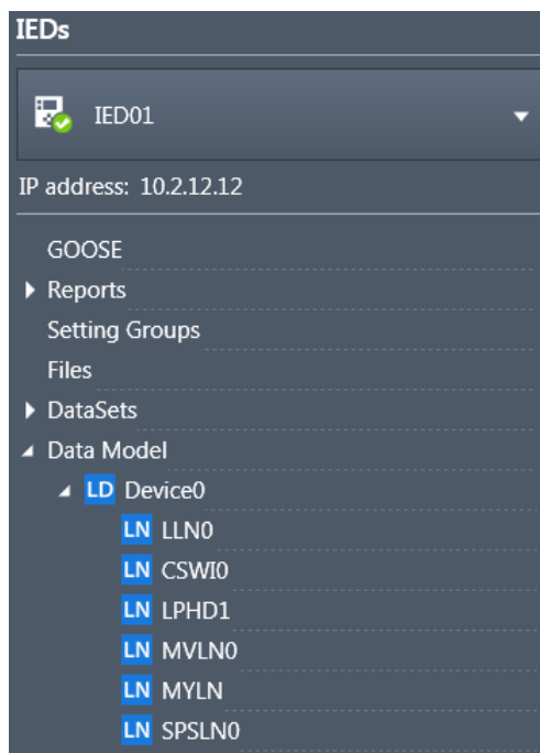
Рисунок 3.22 – Модель данных устройства 61850
