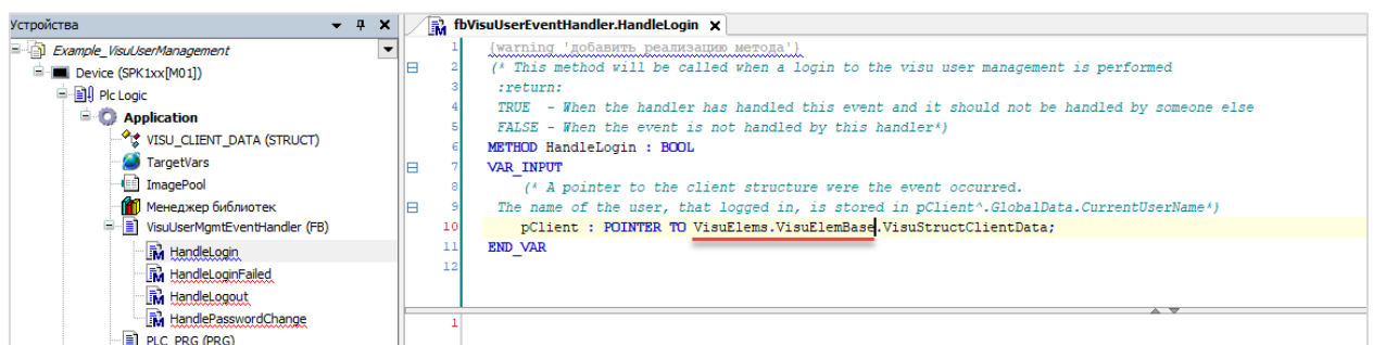
Рисунок 2.9.3 – Указываем пространство имен для структуры VisuStructClientData
