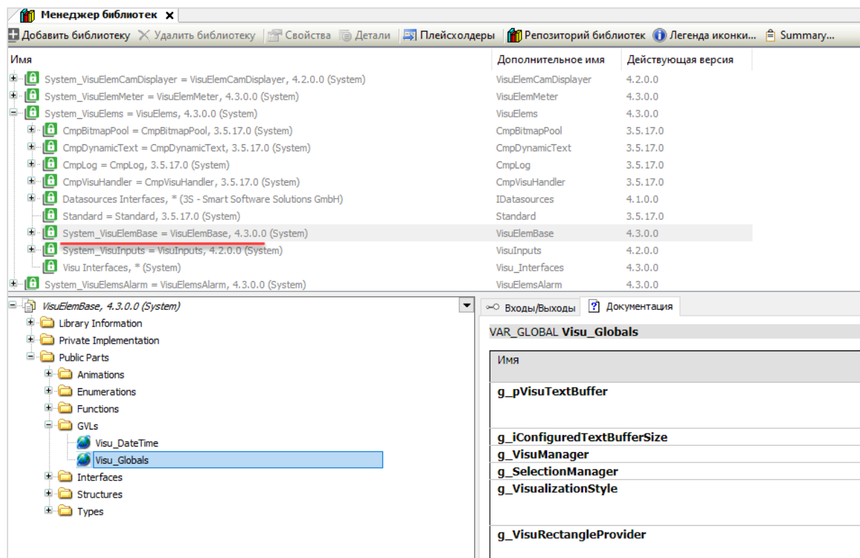
Рисунок 3.1.1 – Структура библиотеки VisuElemBase
