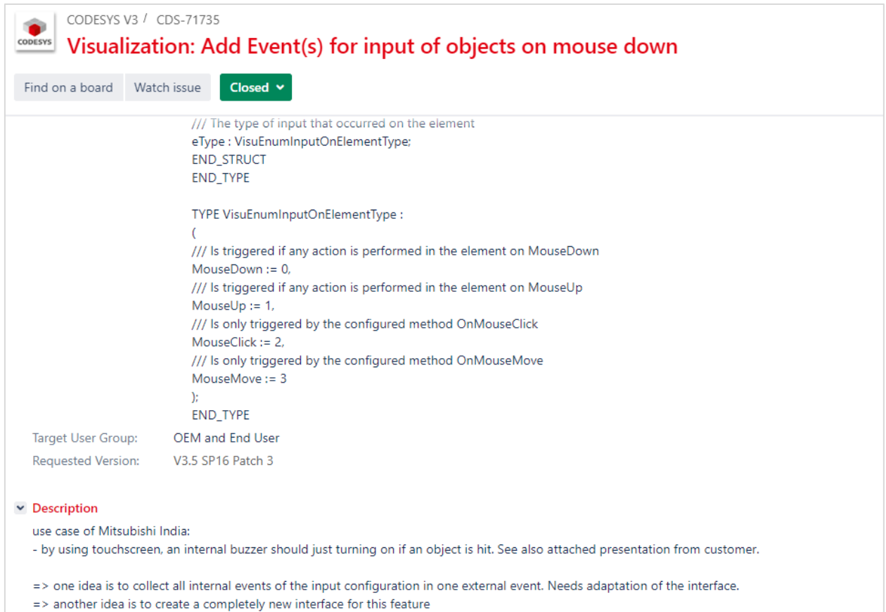
Рисунок 7.4.1.1 – Пожелание в баг-трекере CODESYS, приведшее к появлению интерфейса IInputOnElementEventHandler
