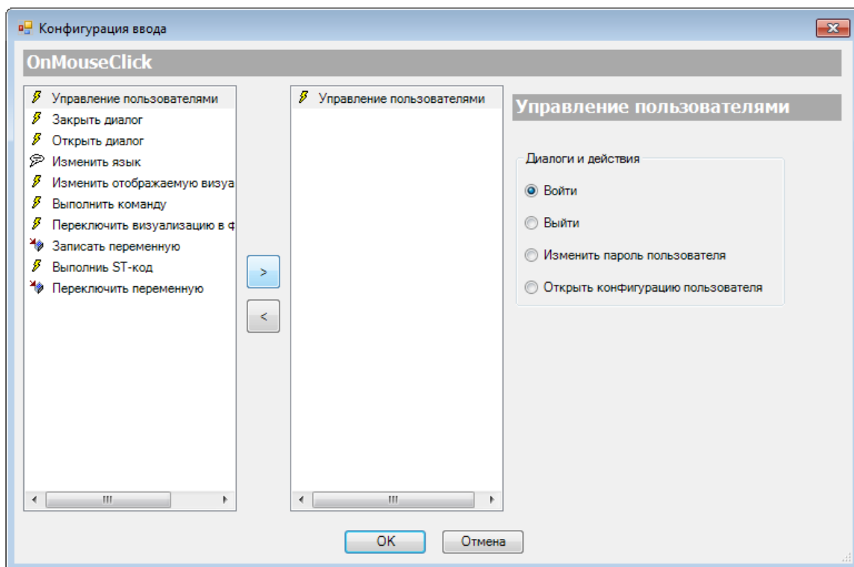
Рисунок 9.3 – Параметры действия Управление пользователями
