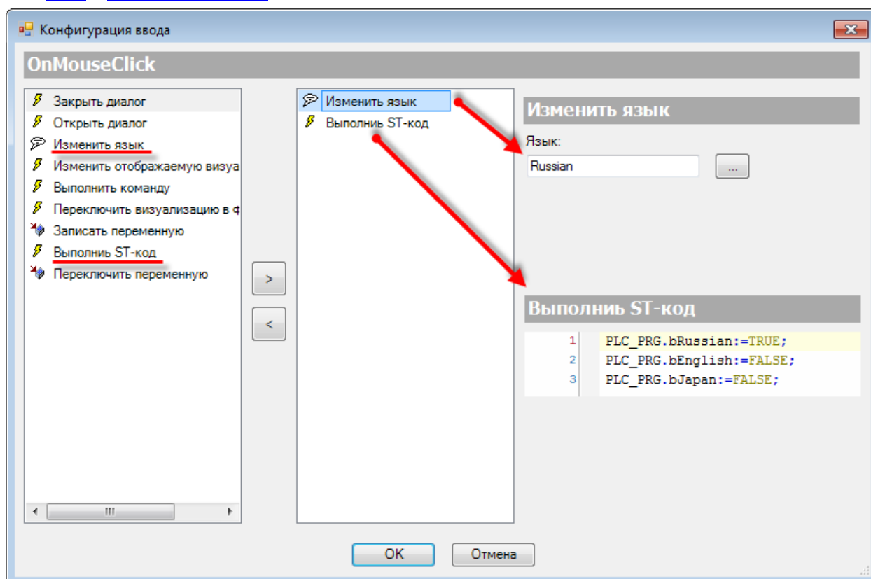
Рисунок 10.343 – Настройки действия кнопки Russian
