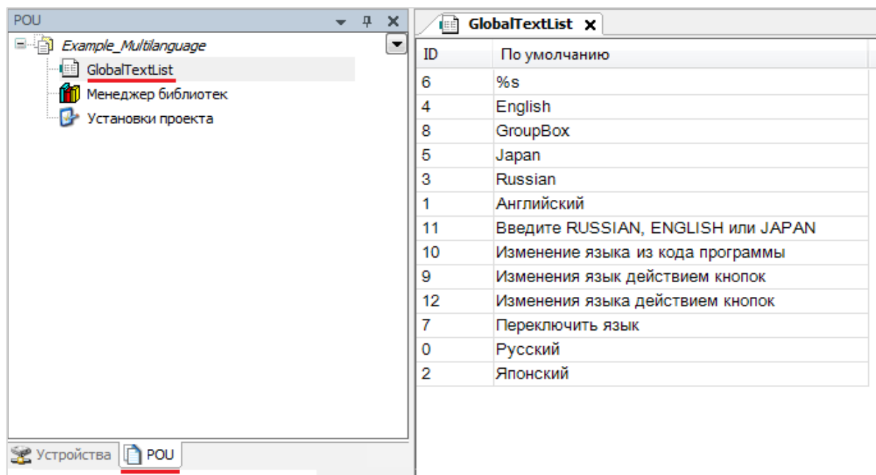
Рисунок 10.354 – Глобальный список текстов проекта
