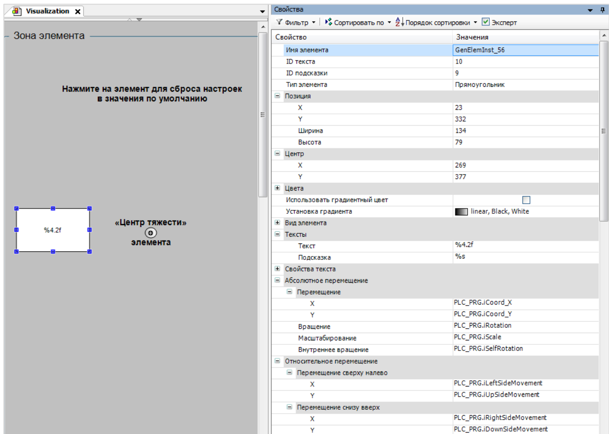
Рисунок 10.15 – Настройки элемента Прямоугольник (начало)
