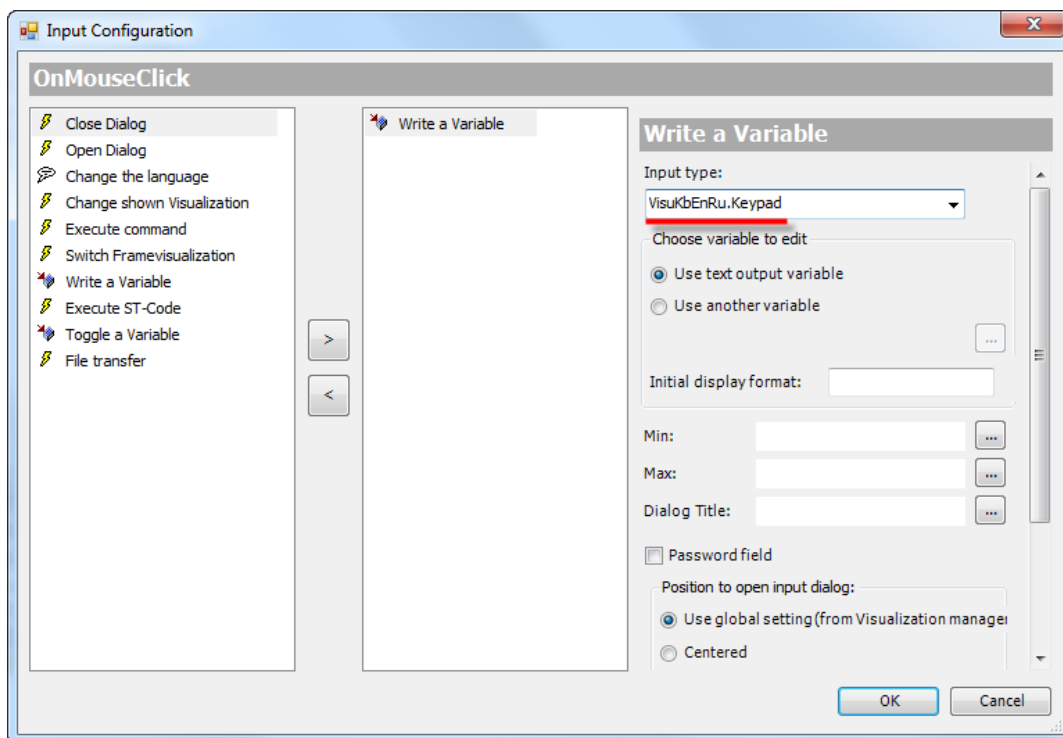
Рисунок 10.434 – Настройки действия кнопки Записать значение
