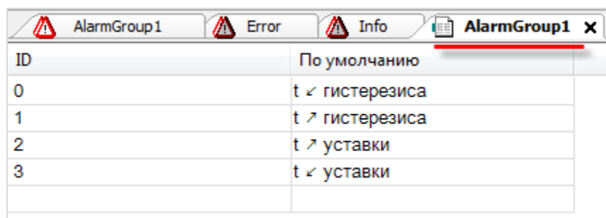
Рисунок 7.98 – Внешний вид Списка текстов тревог
