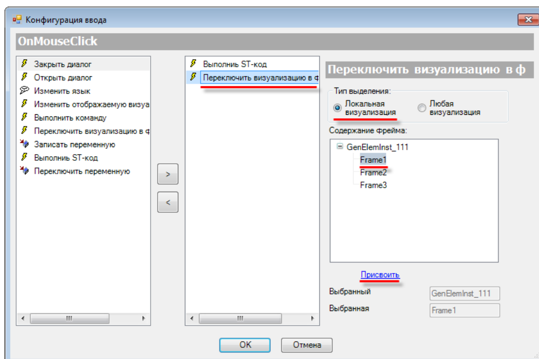
Рисунок 10.400 – Настройка параметра OnMouseClicked кнопки RecipesGroup1, действие Переключить визуализацию во фрейме
