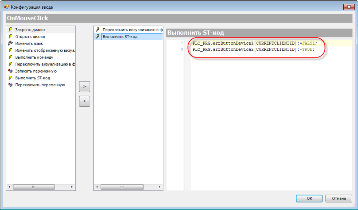
Рисунок 10.472 – Изменение ST-кода кнопки Устройство 2
