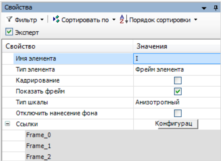
Рисунок 10.71 – Параметры элемента Фрейм
