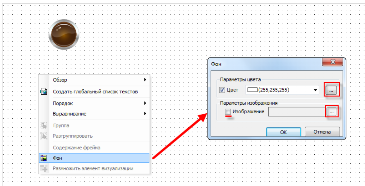
Рисунок 5.9 – Выбор фоновое изображение экрана визуализации
