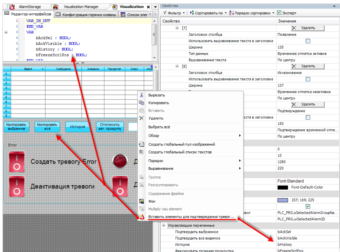
Рисунок 10.249 – Создание кнопок подтверждения тревог
