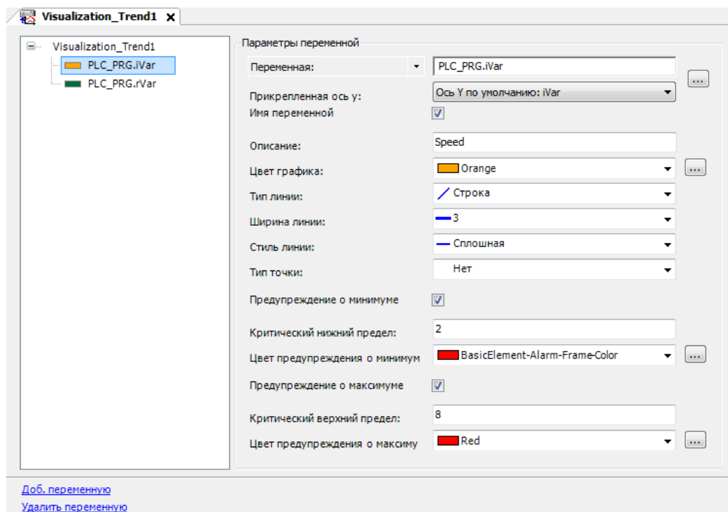
Рисунок 10.166 – Настройки переменной iVar
