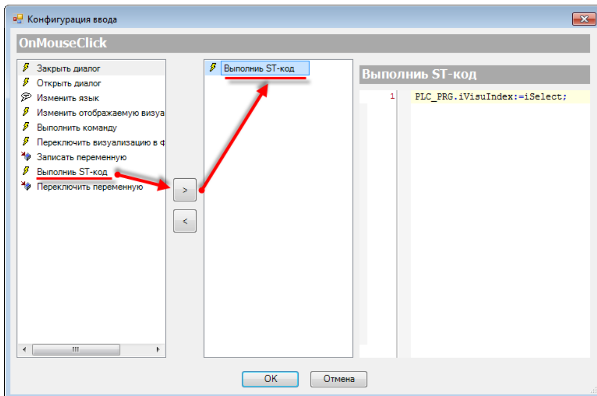
Рисунок 10.279 – Настройки действия кнопки Применить
