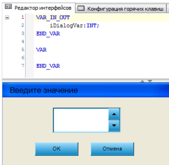
Рисунок 10.289 – Интерфейс и содержимое экрана ChangeValue
