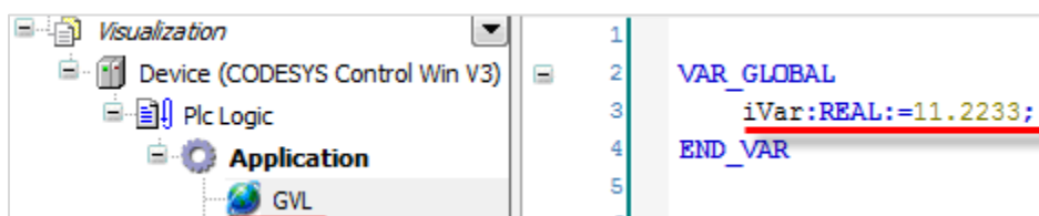
Рисунок 8.3 – Объявление переменной в Глобальном списке переменных
