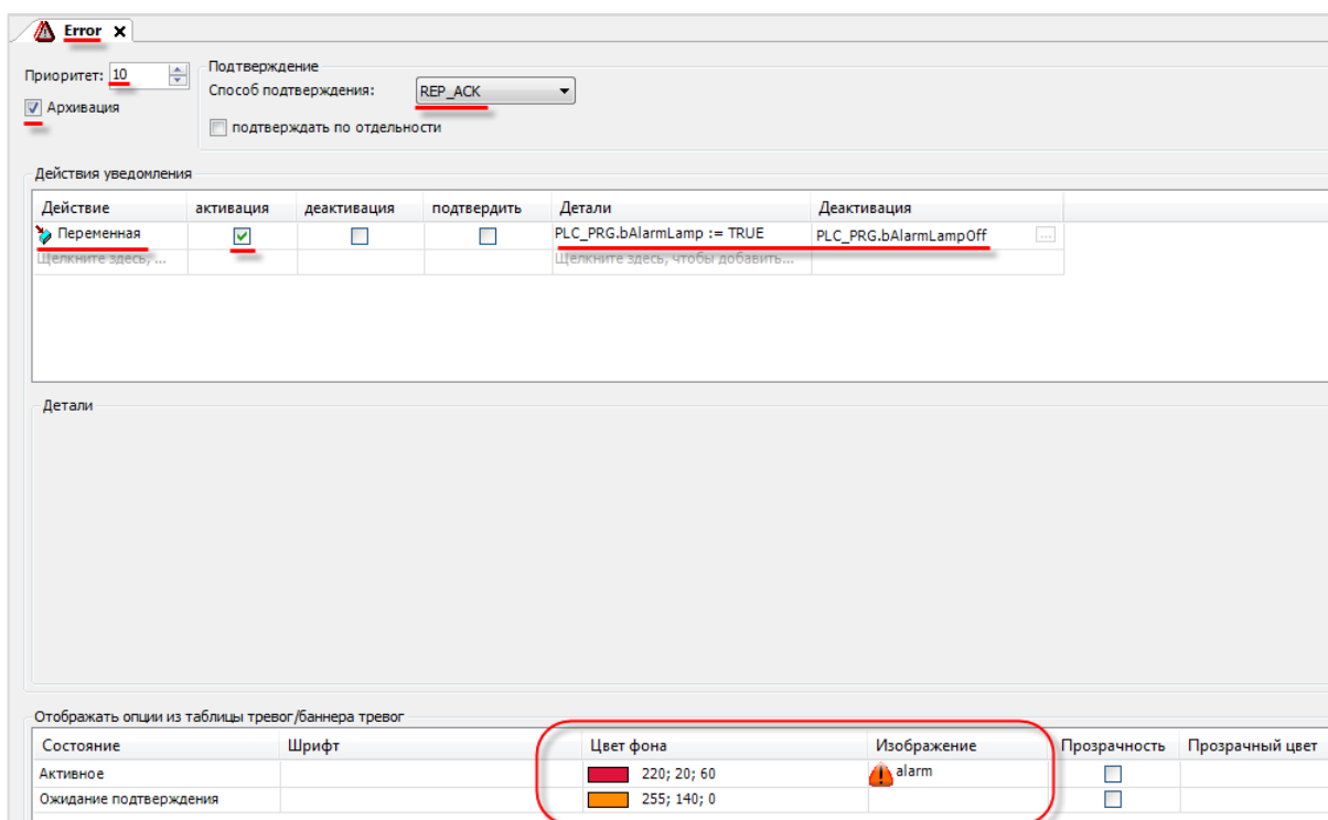
Рисунок 10.242 – Настройки класса тревог Error
