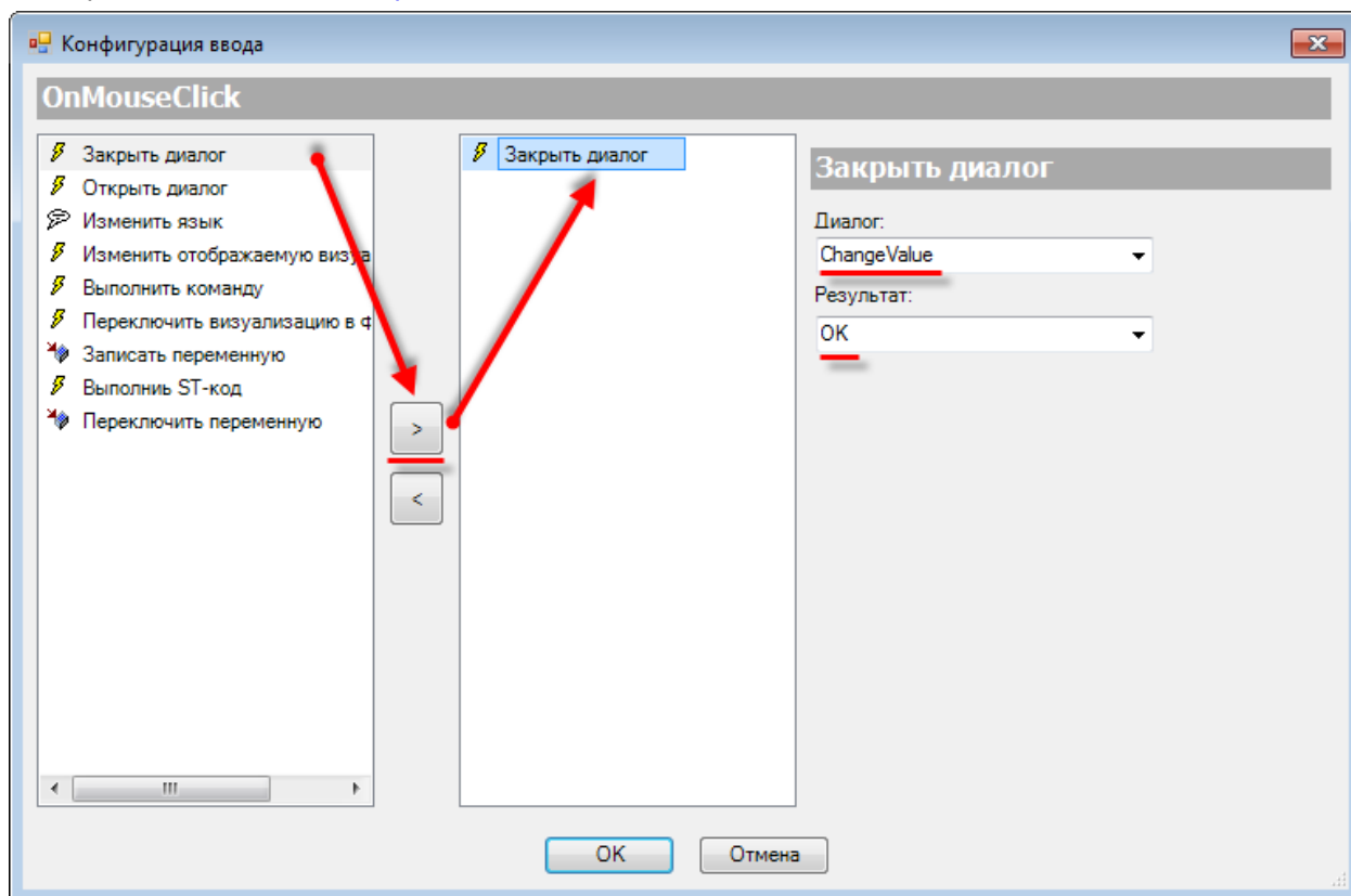
Рисунок 10.292 – Настройки действия кнопки ОК
