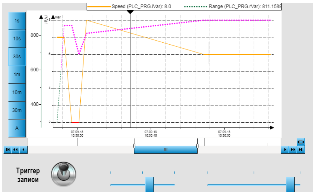
Рисунок 10.182 – Внешний вид тренда (масштаб времени = 30 с)
