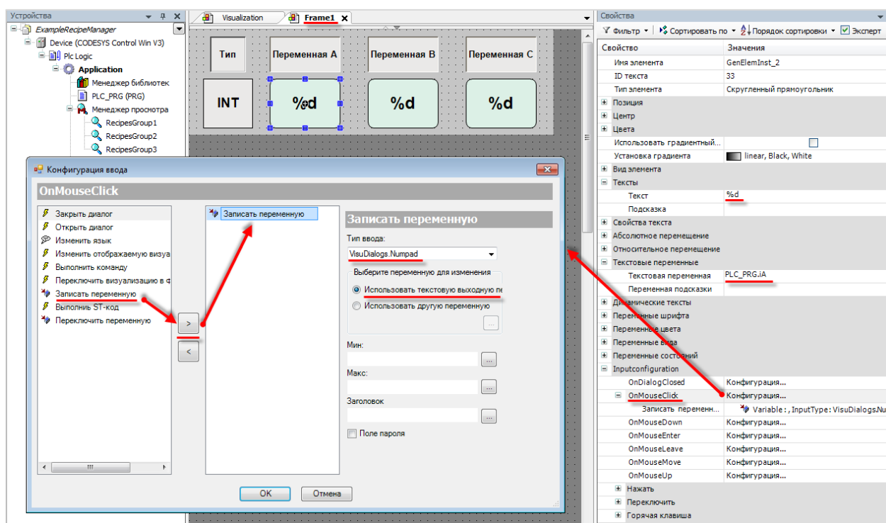
Рисунок 10.394 – Настройка полей вывода переменных типа INT
