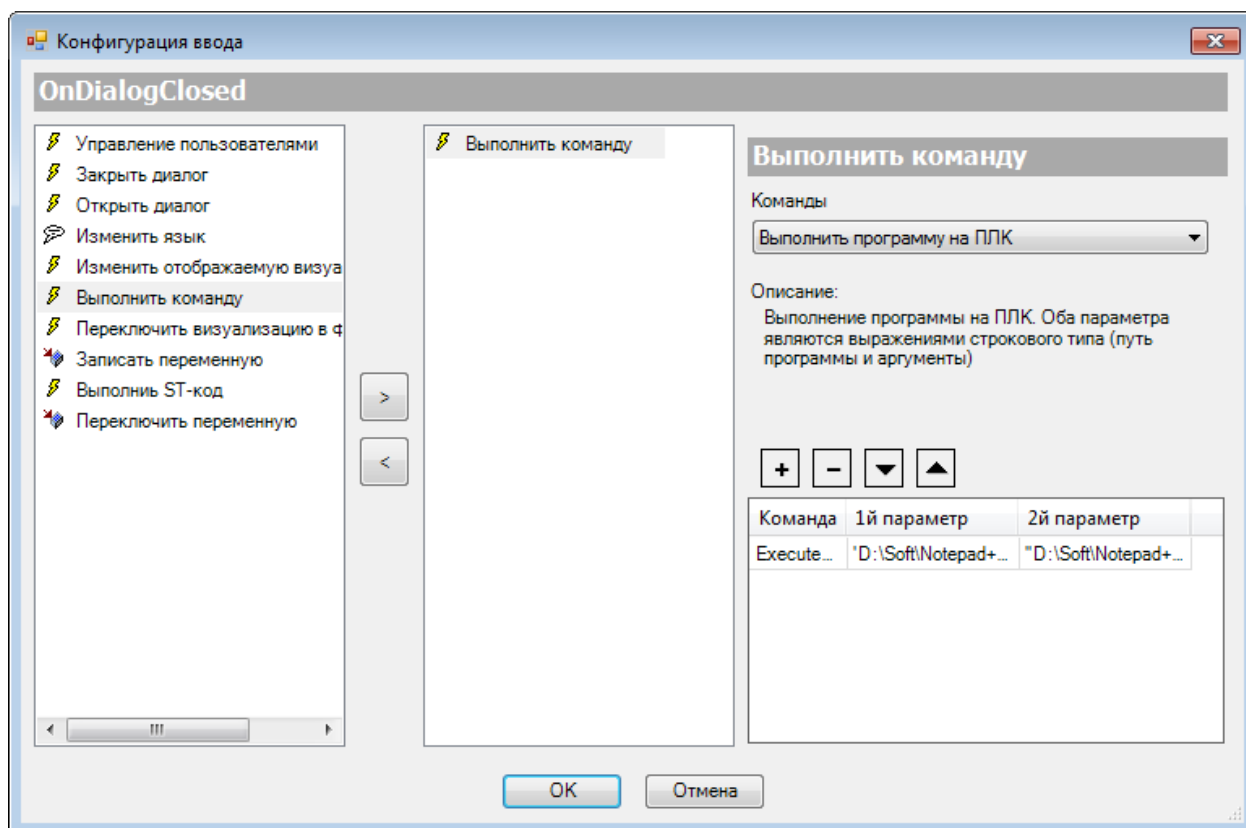
Рисунок 9.11 – Параметры действия Выполнить команду
