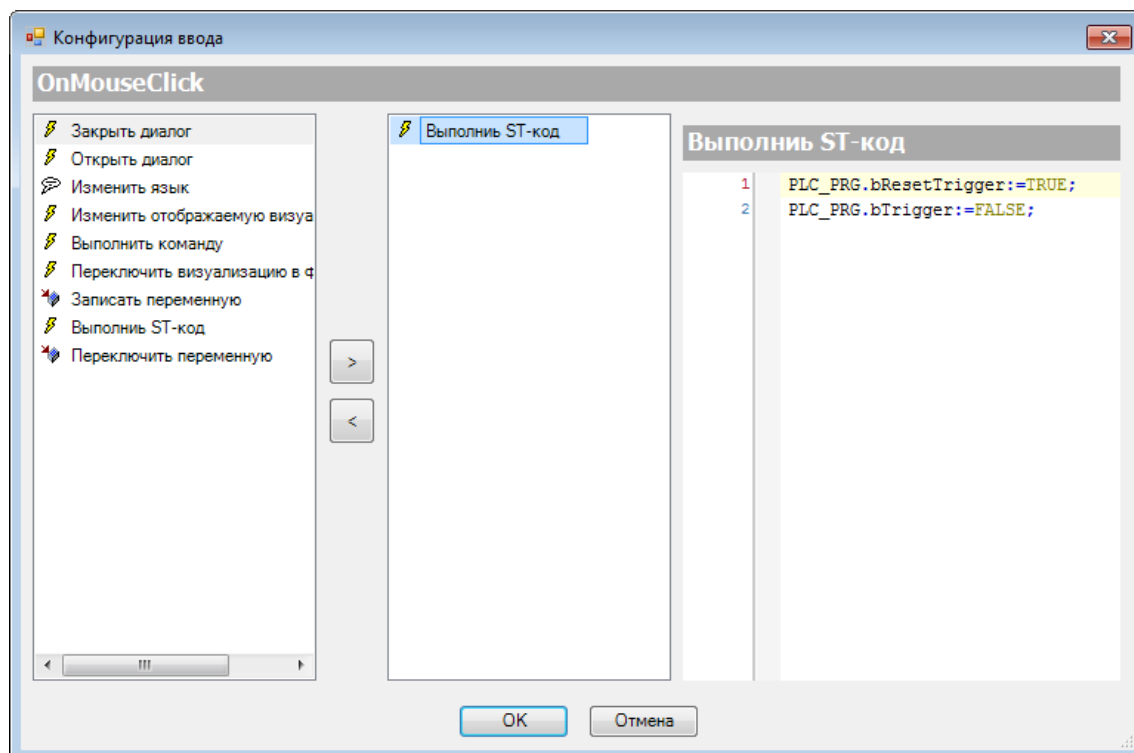
Рисунок 10.157 – ST-код кнопки Сброс триггера
