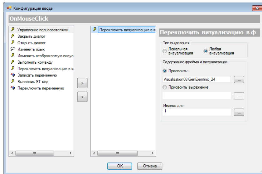
Рисунок 9.12 – Параметры действия Переключить визуализацию во фрейме
