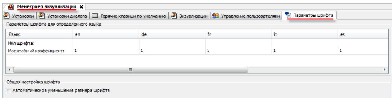
Рисунок 3.7 – Менеджер визуализации, вкладка Установки списков текстов
