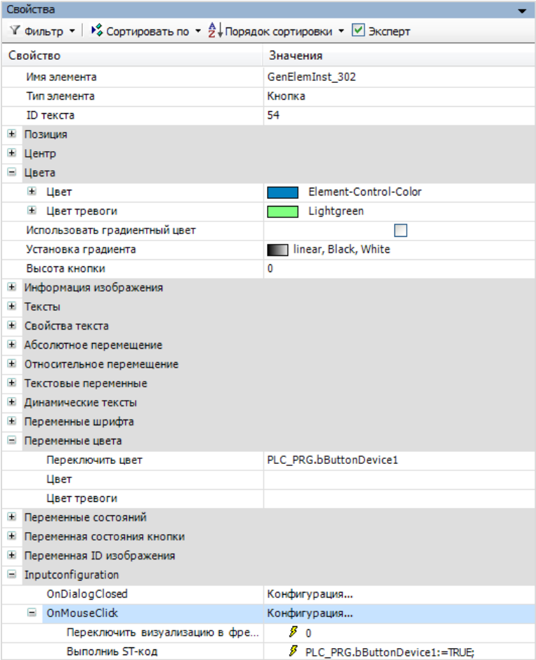
Рисунок 10.307 – Параметры кнопки Устройство 1
