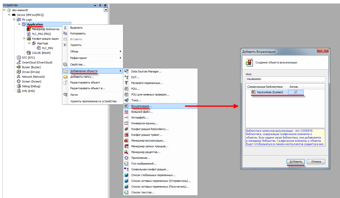
Рисунок 10.475 – Включение поддержки библиотеки VisuSymbols
