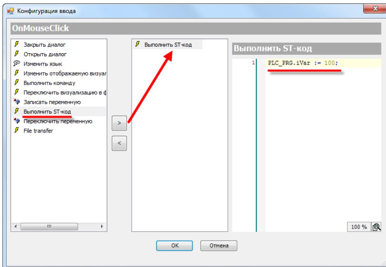
Рисунок 9.15 – Параметры действия Выполнить ST-код
