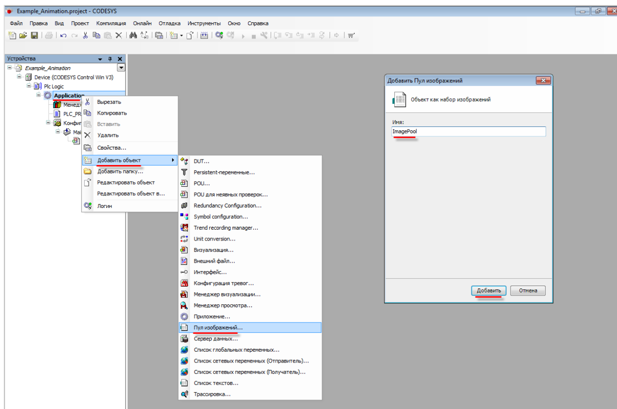
Рисунок 10.318 – Добавление в проект пула изображений
