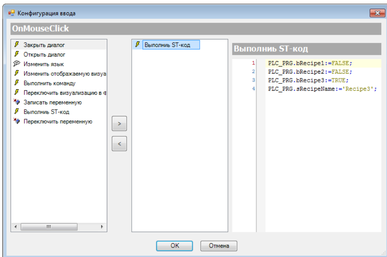
Рисунок 10.406 – Настройка параметра OnMouseClicked кнопки Recipe3, действие Выполнить ST-код
