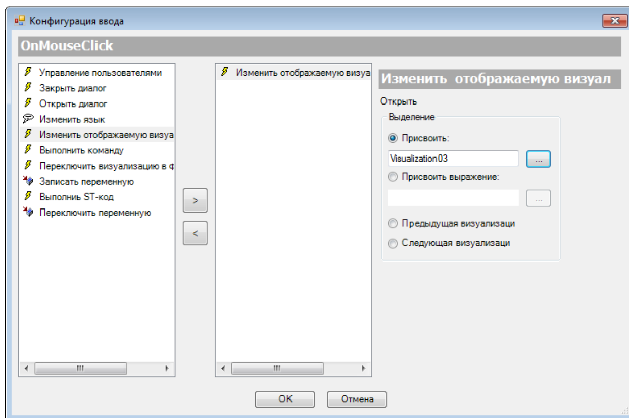
Рисунок 9.10 – Параметры действия Изменить отображаемую визуализацию
