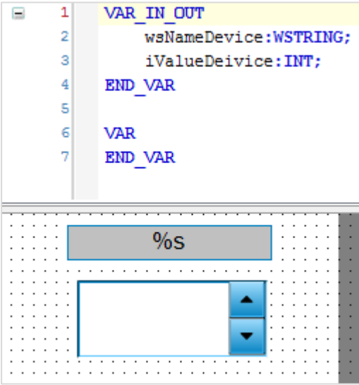
Рисунок 10.302 – Интерфейс и содержимое экрана Frame
