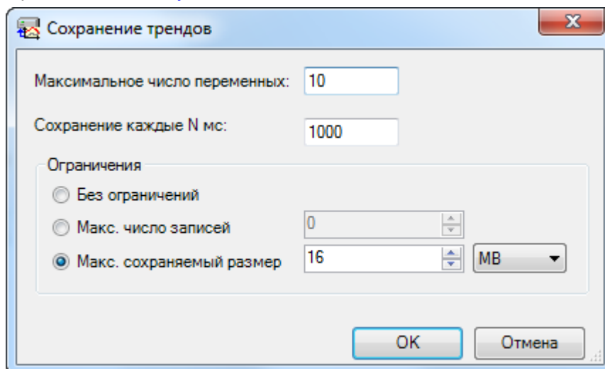
Рисунок 7.71 – Конфигурация тренда – Сохранение трендов
