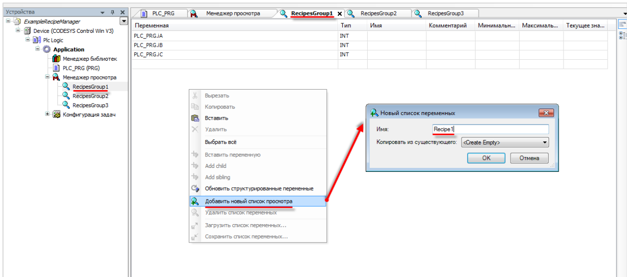
Рисунок 10.387 – Создание рецепта в группе рецептов
