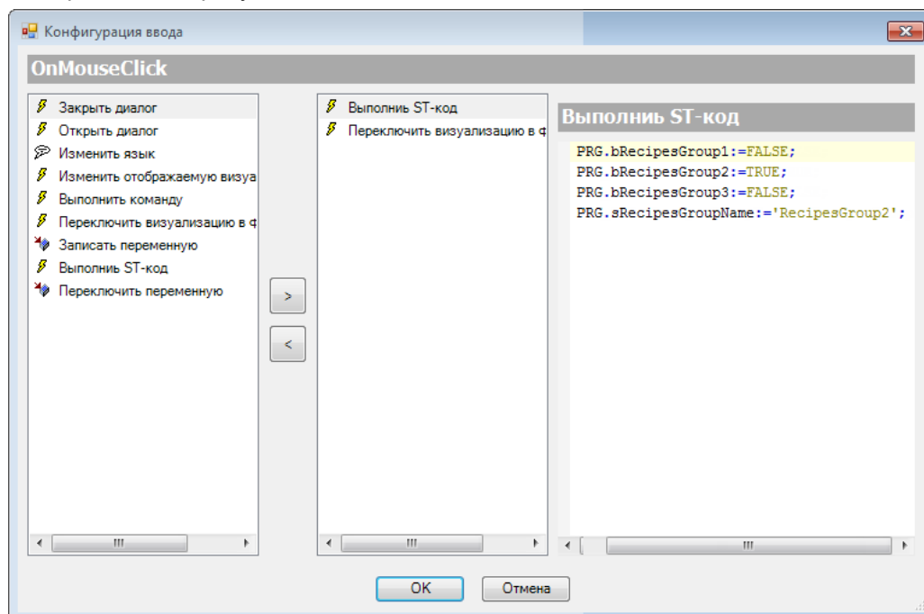
Рисунок 10.401 – Настройка параметра OnMouseClicked кнопки RecipesGroup2, действие Выполнить ST-код
