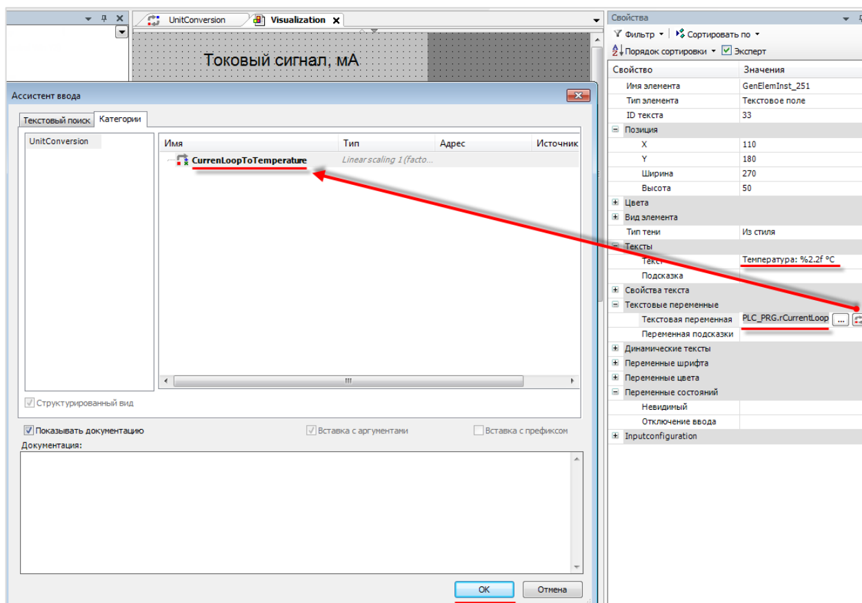
Рисунок 10.423 – Выбор шаблона преобразования для элемента Текстовое поле
