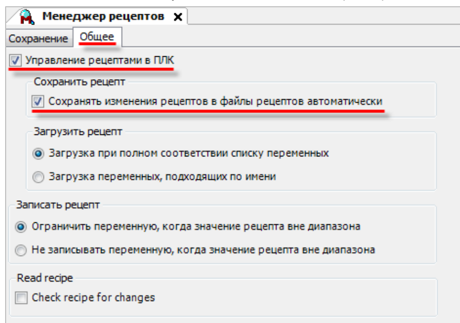
Рисунок 10.383 – Настройки Менеджера рецептов, вкладка Общее
