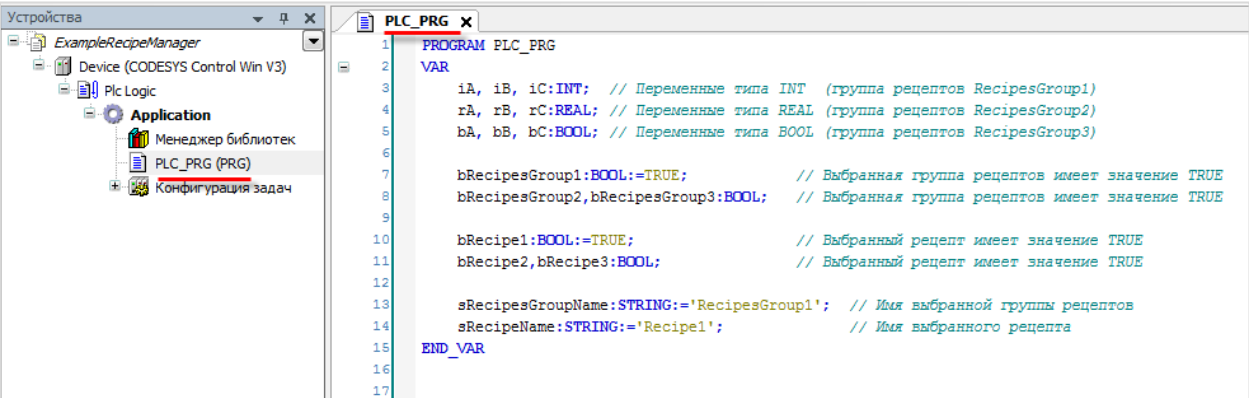
Рисунок 10.380 – Объявление переменных в программе PLC_PRG
