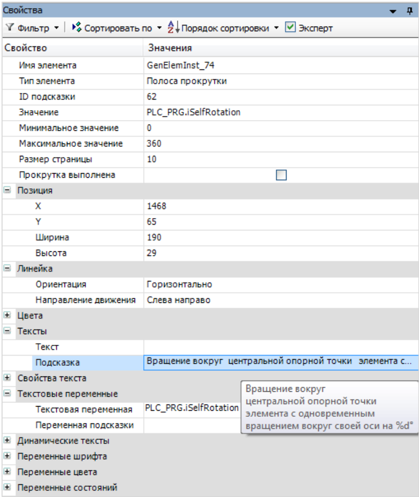
Рисунок 10.25 – Настройки элемента Полоса прокрутки 2
