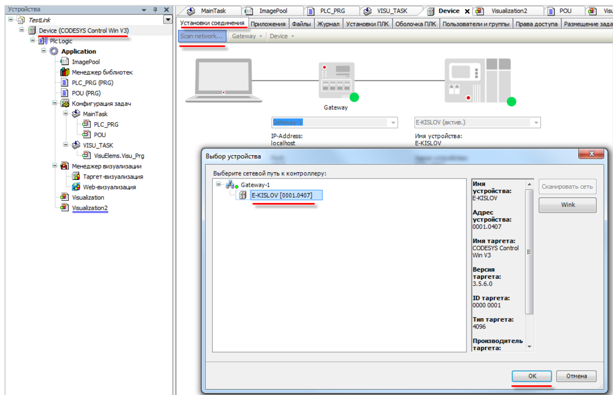
Рисунок 10.2 – Окно сканирования сети. Подключение к виртуальному контроллеру
