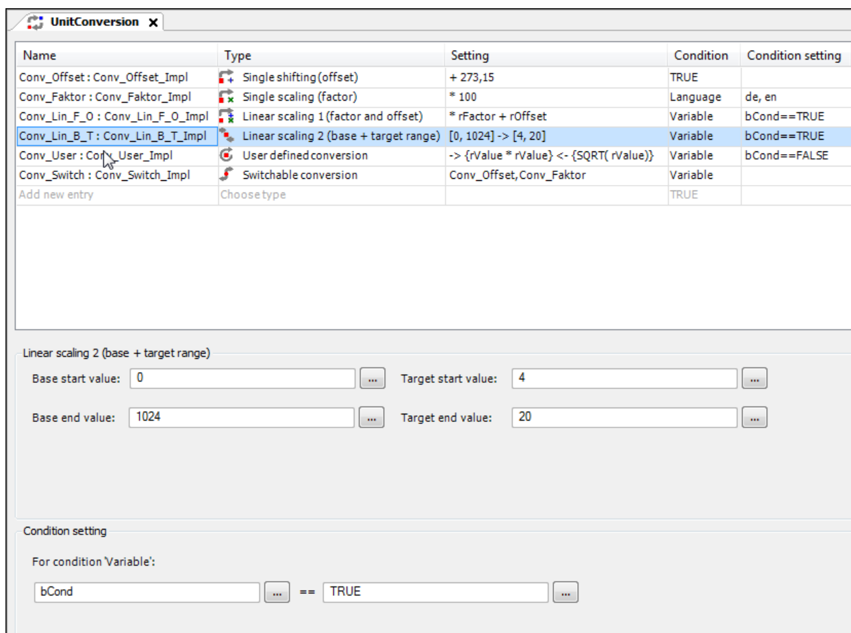
Рисунок 10.417 – Внешний вид компонента Unit Conversion
