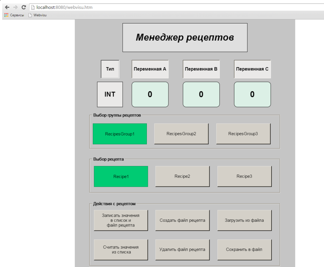
Рисунок 10.415 – Web-визуализация проекта в браузере Chrome
