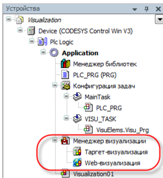
Рисунок 2.3 – Компонент Менеджер визуализации в Панели устройств проекта
