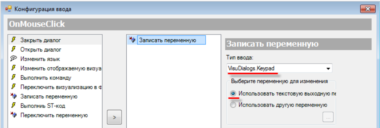
Рисунок 10.75 – Настройки действия кнопки Выбран фрейм
