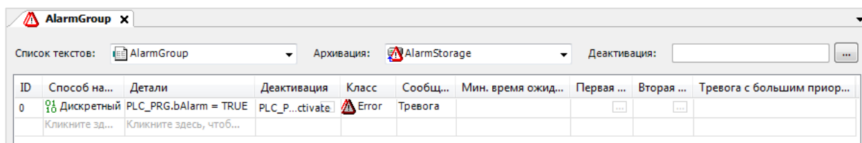
Рисунок 7.97 – Настройки группы тревог AlarmGroup
