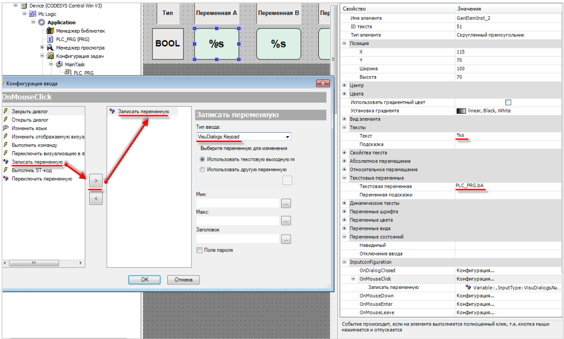
Рисунок 10.396 – Настройка полей вывода переменных типа BOOL
