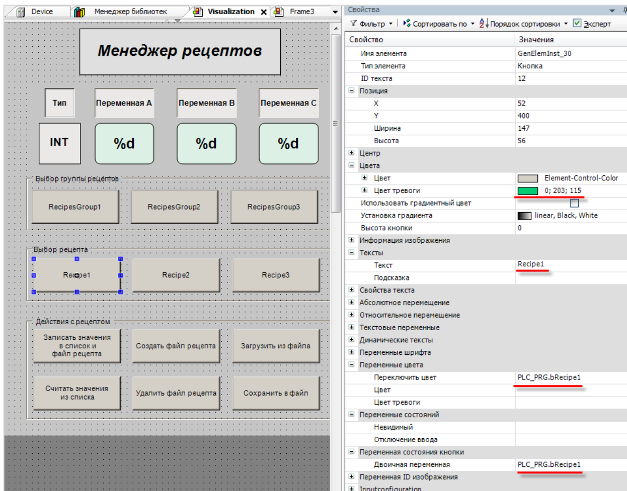
Рисунок 10.403 – Настройки кнопки выбора рецепта Recipe1
