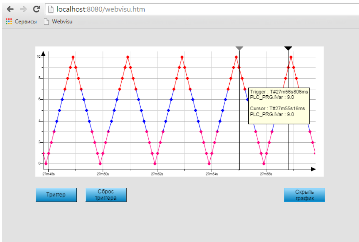
Рисунок 10.161 – Web-визуализация проекта в браузере Chrome
