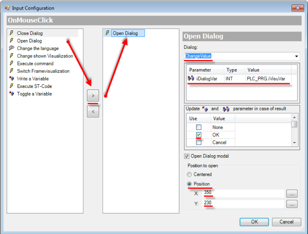
Рисунок 10.295 – Настройки действия кнопки Изменить значение
