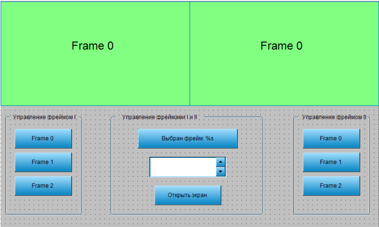
Рисунок 10.72 – Экран визуализации Visu (фреймы сконфигурированы)
