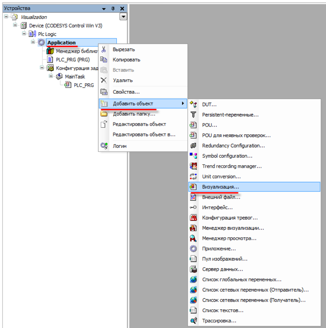
Рисунок 2.1 – Добавление экрана визуализации в проект
