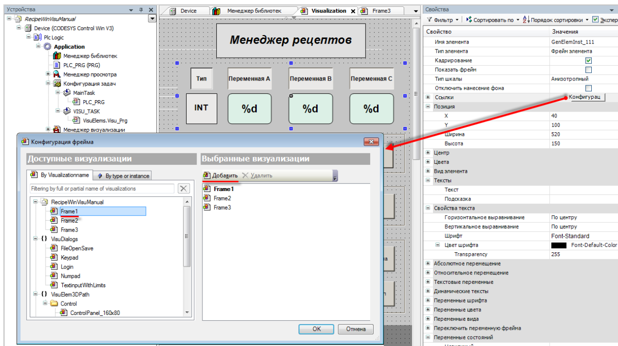
Рисунок 10.397 – Настройка содержимого элемента Фрейм
