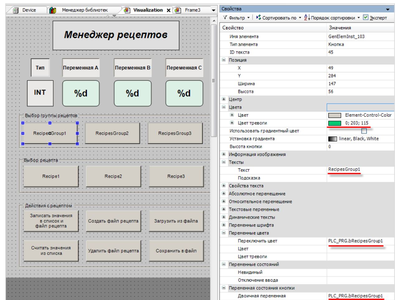
Рисунок 10.398 – Настройки кнопки выбора групп рецептов RecipesGroup1
