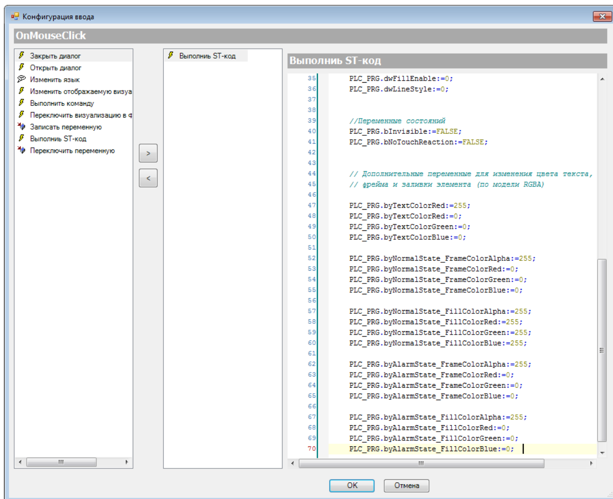
Рисунок 10.19 – Настройки параметра OnMouseClicked вкладки InputConfiguration элемента Прямоугольник (окончание)
