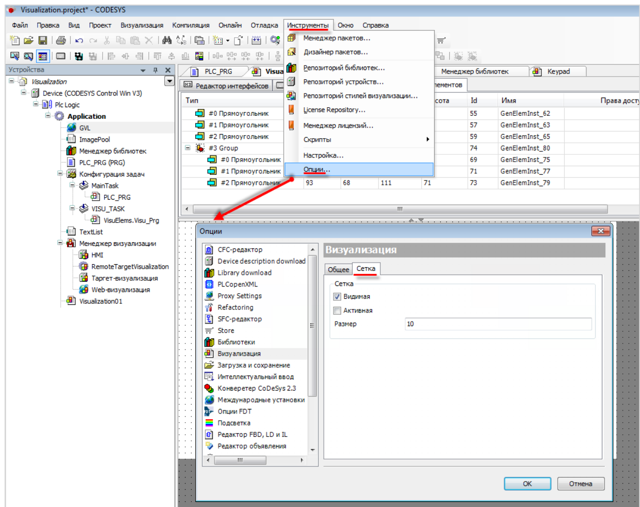
Рисунок 5.13 – Настройки сетки редактора визуализации
