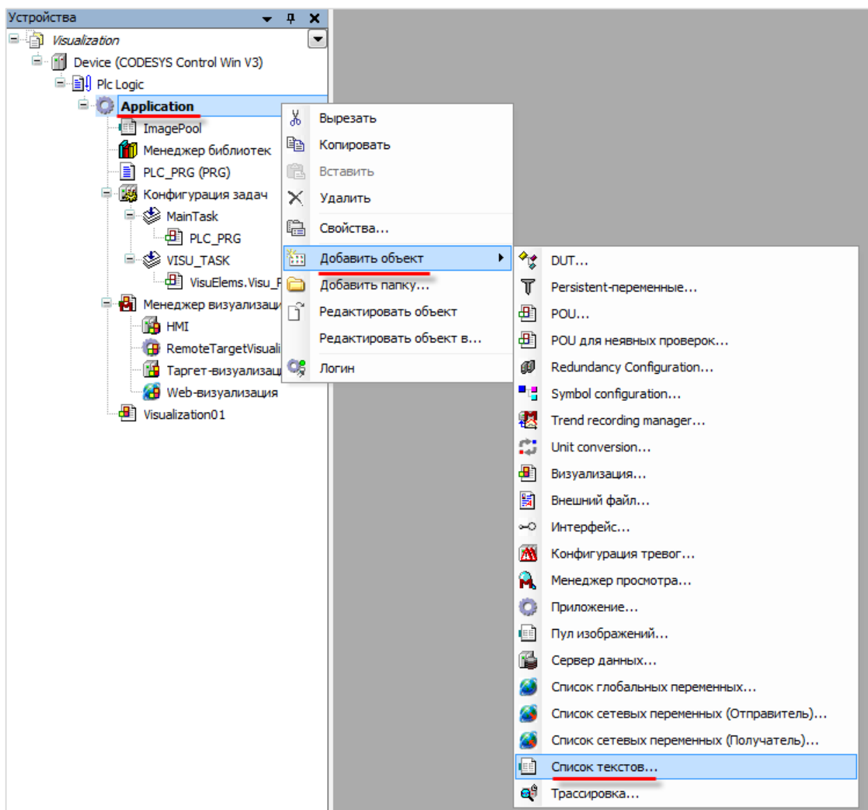
Рисунок 6.4 – Добавление Списка текстов в проект
