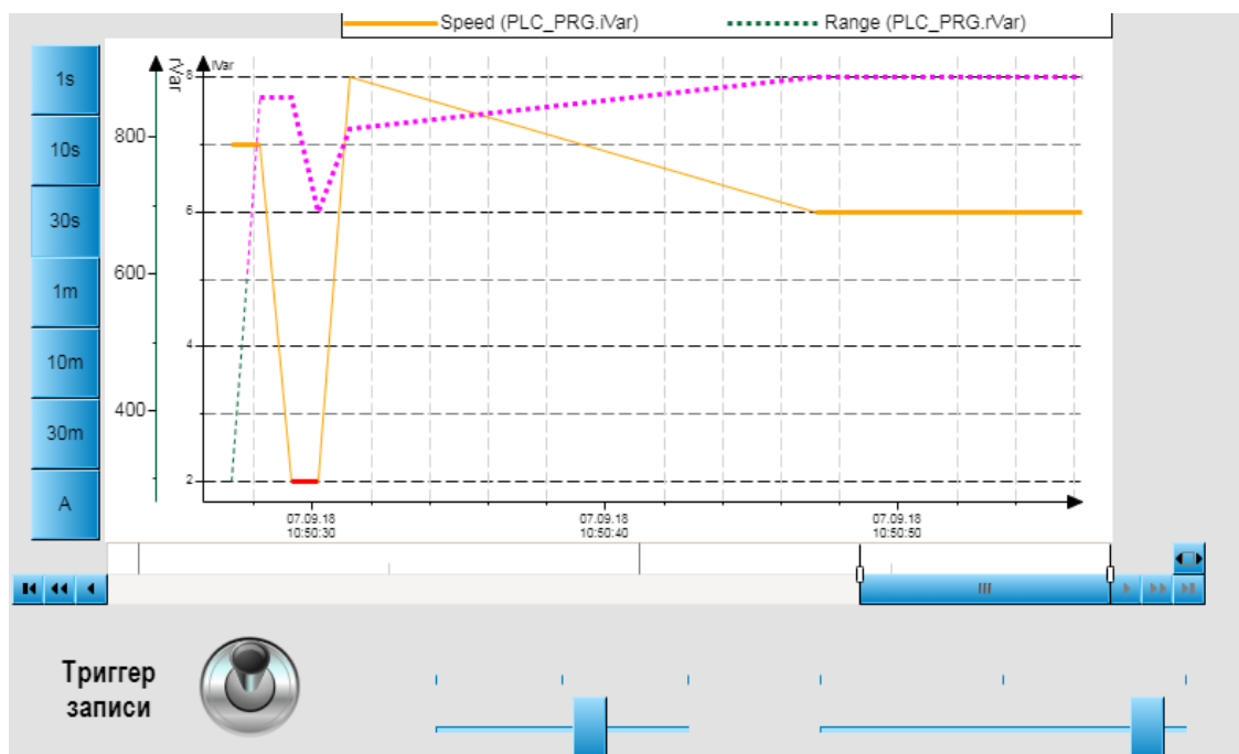
Рисунок 10.181 – Внешний вид тренда после включения и отключения триггера записи
