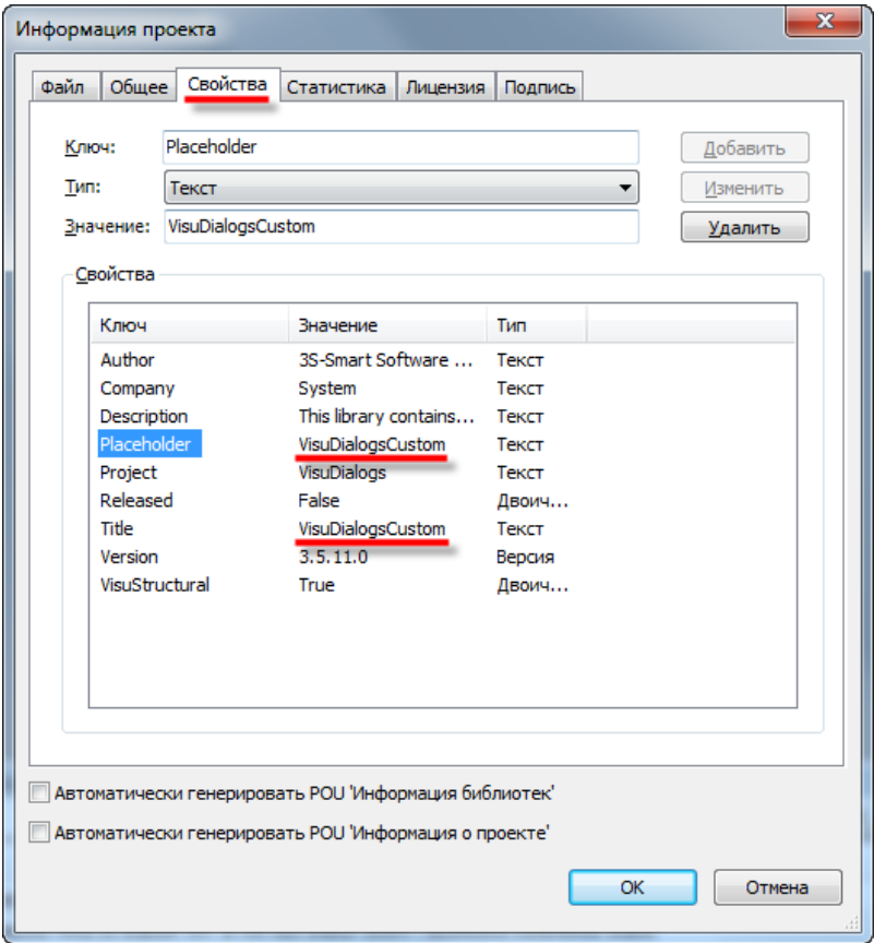
Рисунок 10.478 – Изменение ключей библиотеки
