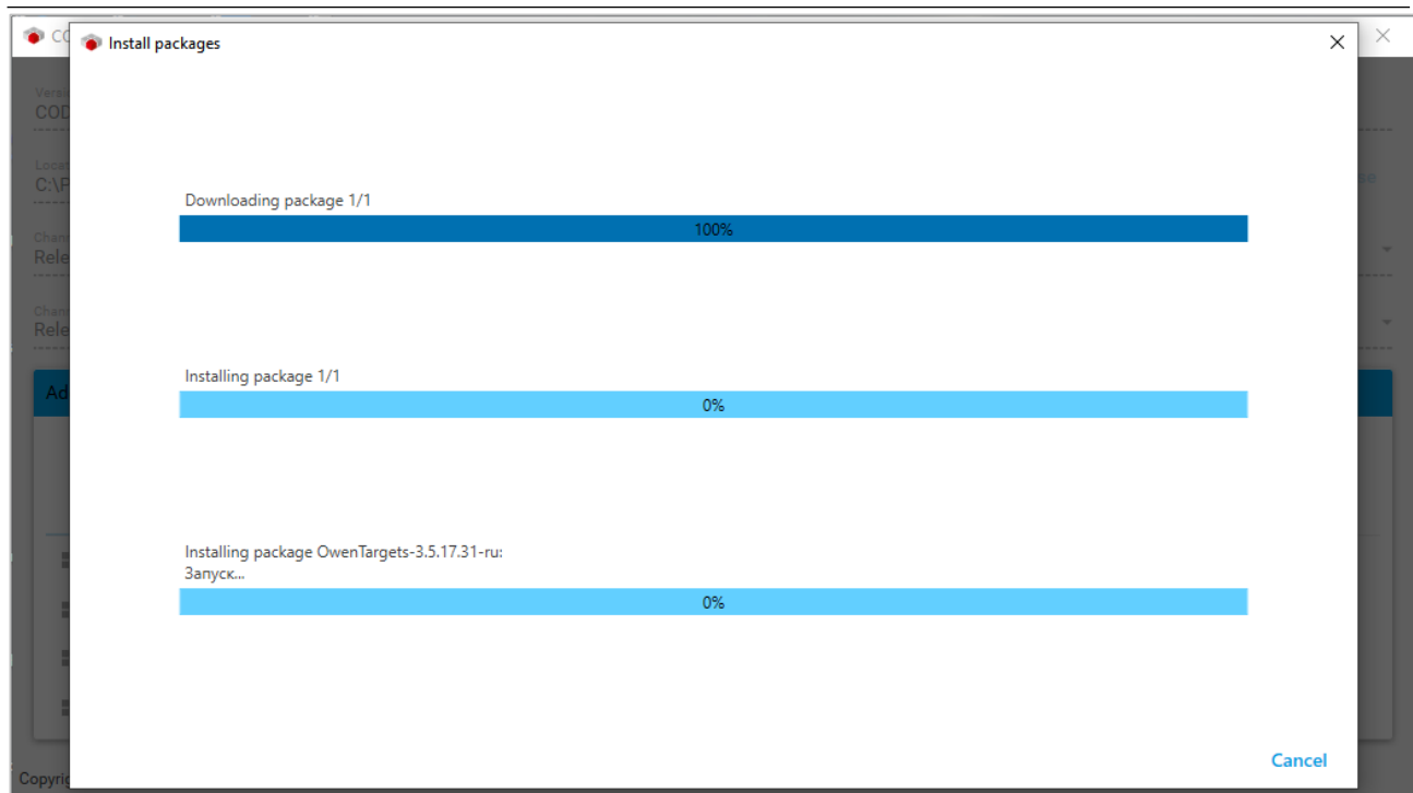
Рисунок 2.6 – Установка пакета
