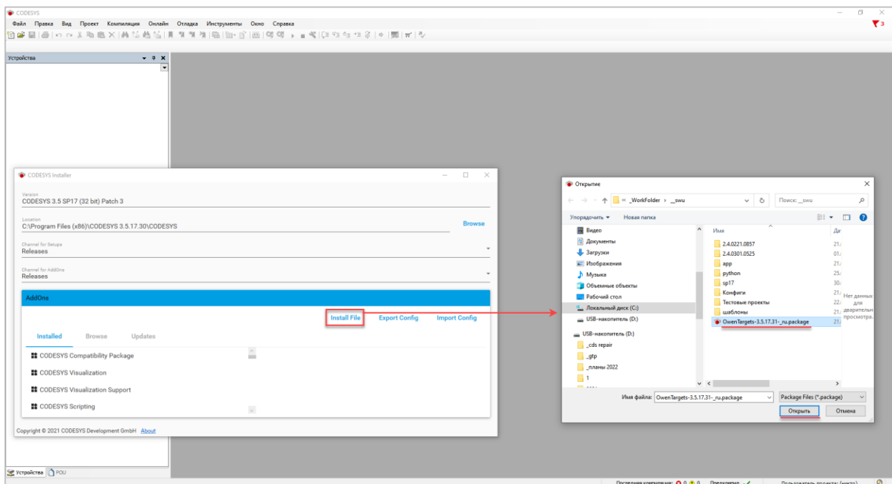
Рисунок 2.2 – Выбор пакета
