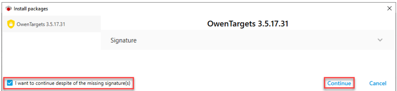
Рисунок 2.4 – Подтверждение установки (2)
