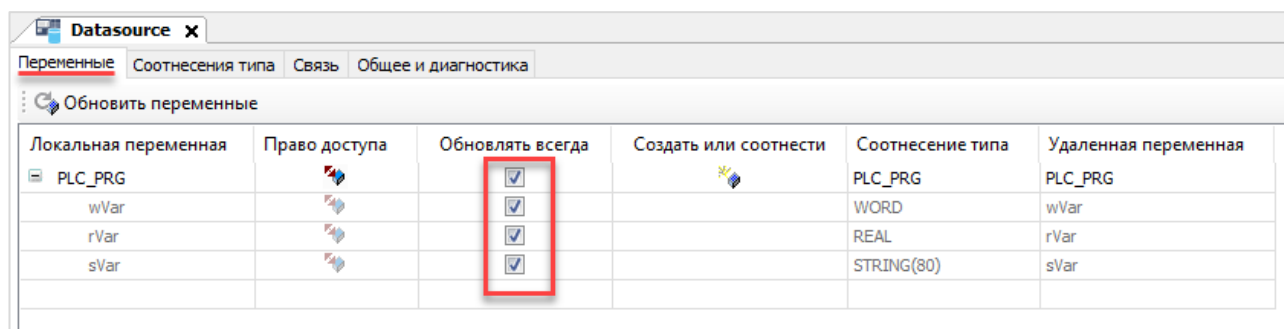
Рисунок 3.2.12 – Настройки источника данных, вкладка Переменные
