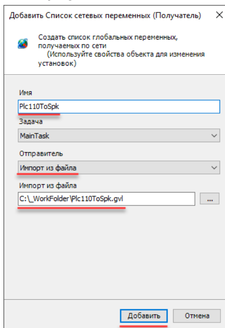
Рисунок 2.5.11 – Импорт списка сетевых переменных
