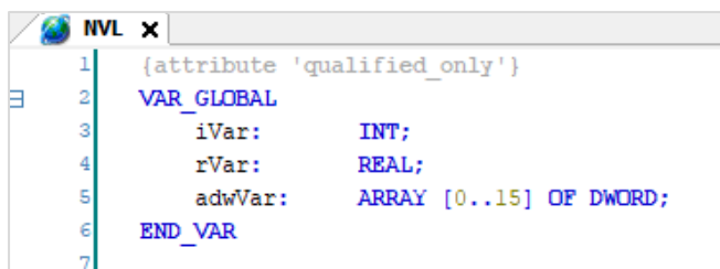
Рисунок 2.2.4 – Объявление сетевых переменных
