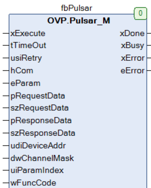
Рисунок 2.12.1 – Внешний вид ФБ Pulsar_M на языке CFC
