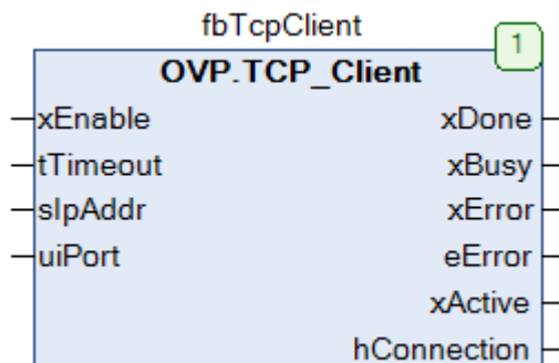
Рисунок 2.3.2 – Внешний вид ФБ TCP_Client на языке CFC
