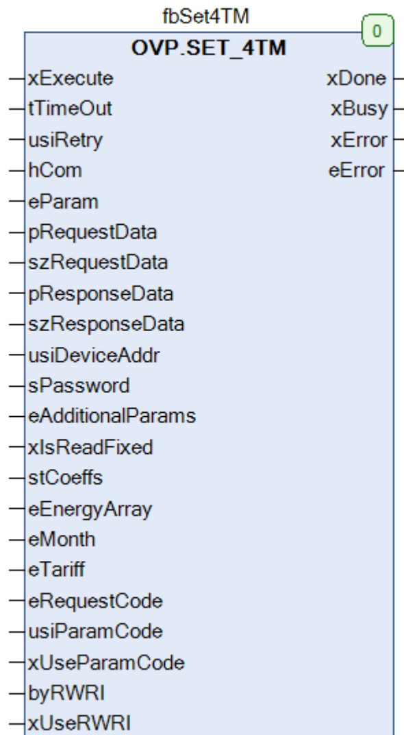
Рисунок 2.11.1 – Внешний вид ФБ SET_4TM на языке CFC
