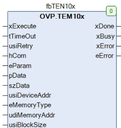
Рисунок 2.4.1 – Внешний вид ФБ TEM10x на языке CFC
