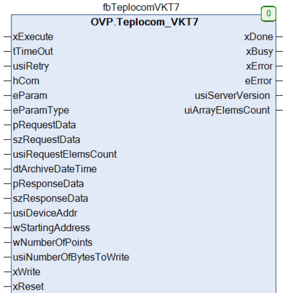
Рисунок 2.10.1 – Внешний вид ФБ Teplocom_VKT7 на языке CFC
