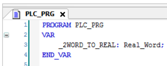
Рисунок А.3 – Объявление экземпляра объединения в программе
