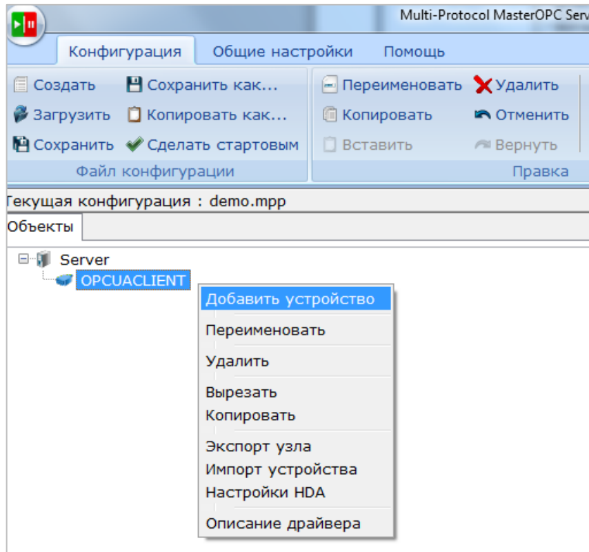
Рисунок 4.6.2 – Добавление устройства
