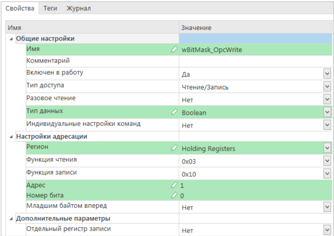
Рисунок 4.5.4 – Настройки тега wBitMask_OpcWrite
