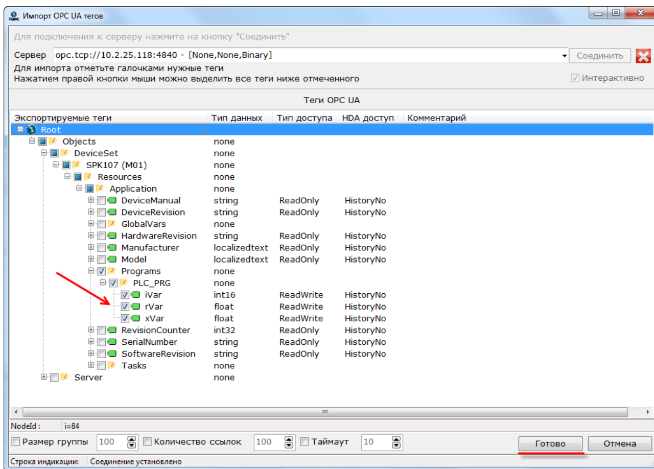
Рисунок 4.6.9 – Выбор тегов
