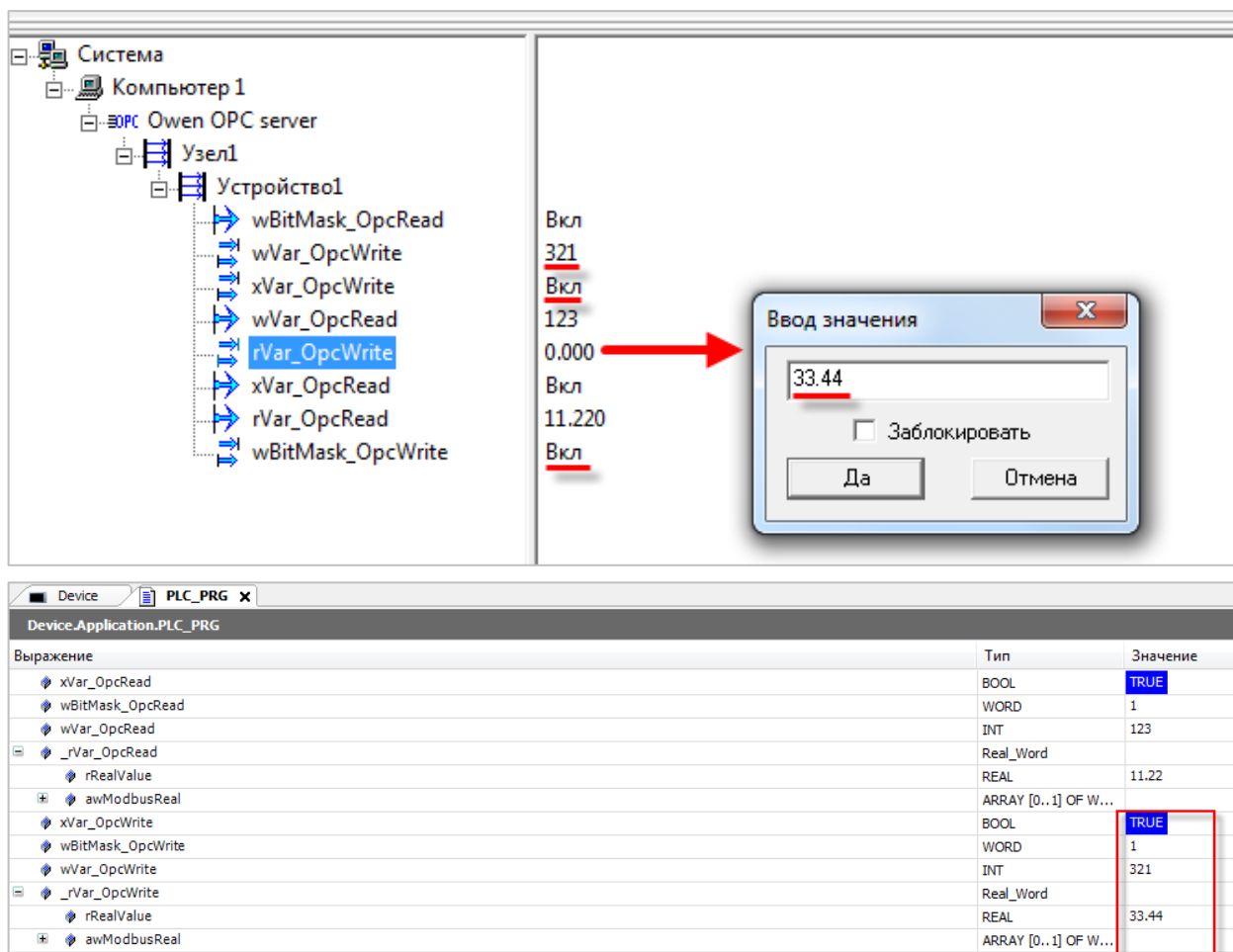
Рисунок 4.7.7 – Запись данных из MasterSCADA в контроллер
