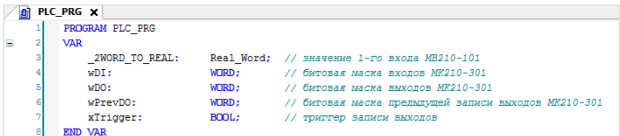
Рисунок 4.11.5 – Объявление переменных программы
