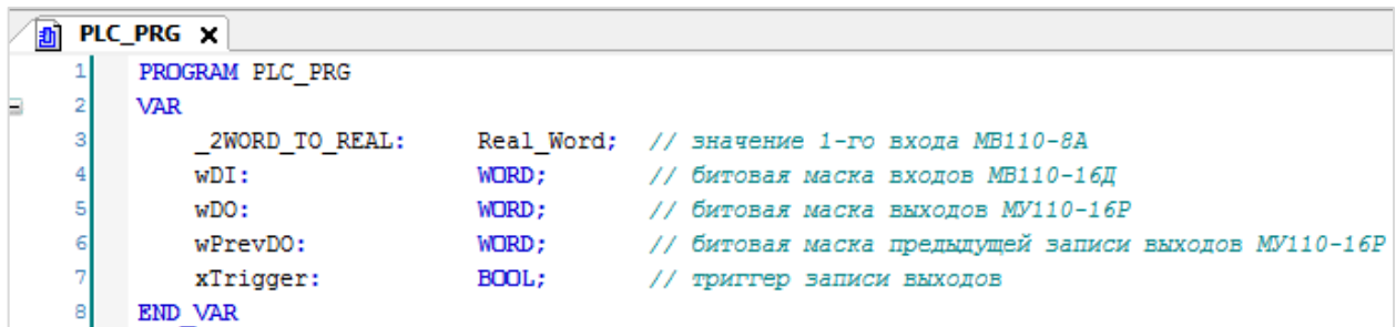
Рисунок 4.9.5 – Объявление переменных программы
