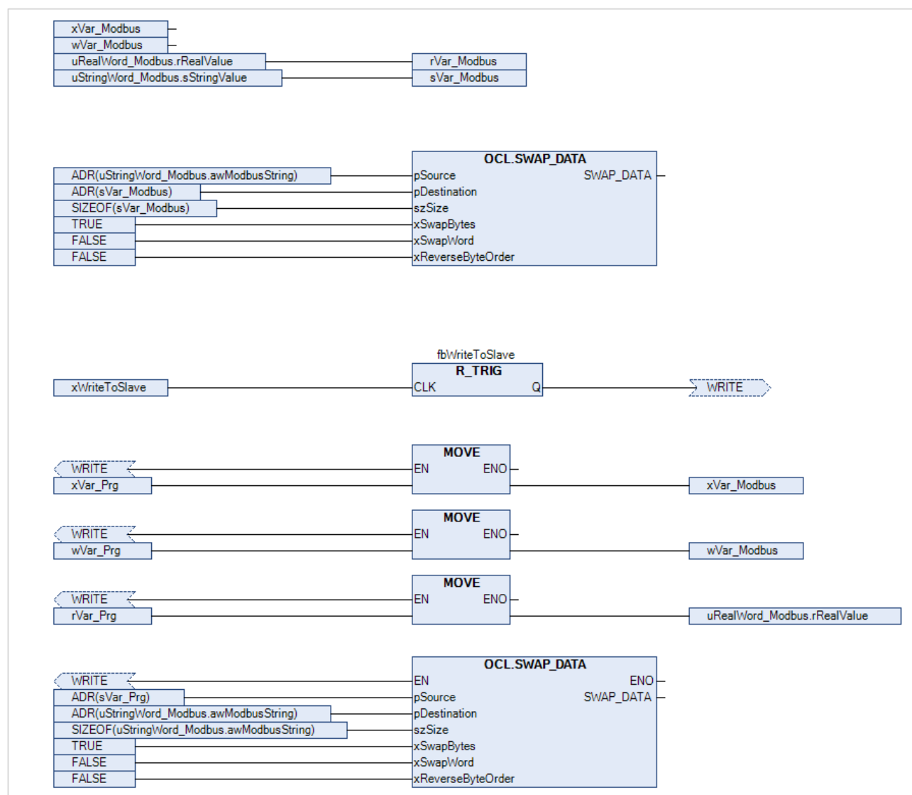
Рисунок 4.10.7 – Код программы PLC_PRG
