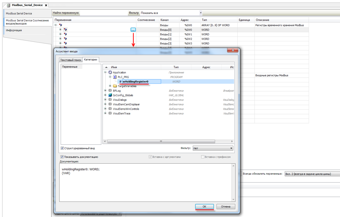
Рисунка 4.3.6 – Привязка переменных программы к регистрам Modbus RTU Slave
