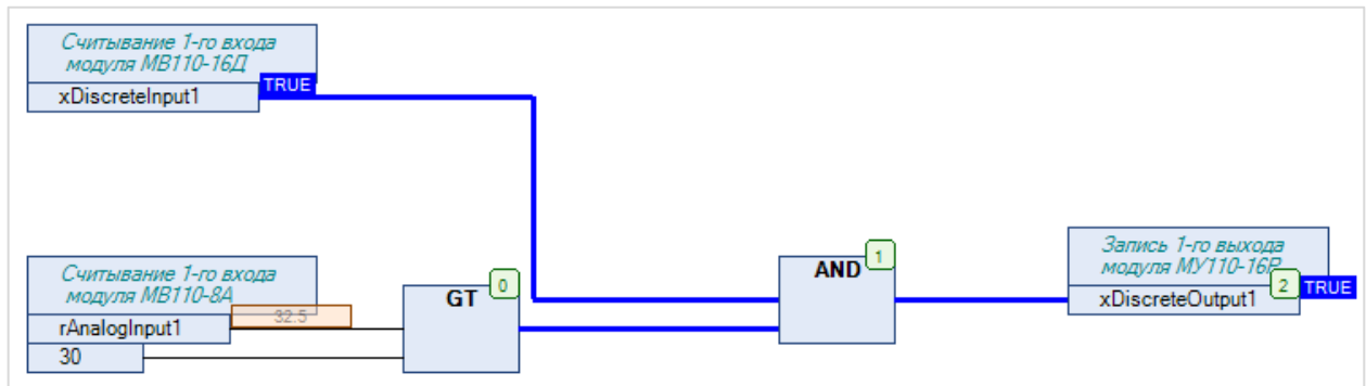
Рисунок 3.2.16 – Выполнение программы в режиме Online
