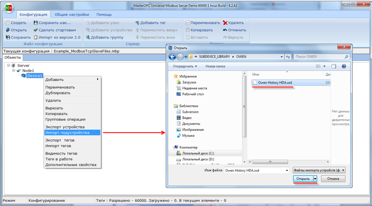
Рисунок 5.9.51 – Импорт подустройства
