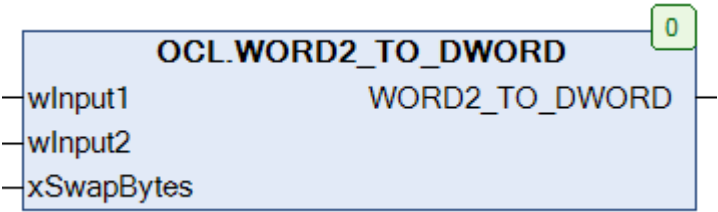
Рисунок 5.8.5 – Внешний вид функции WORD2_TO_DWORD на языке CFC
