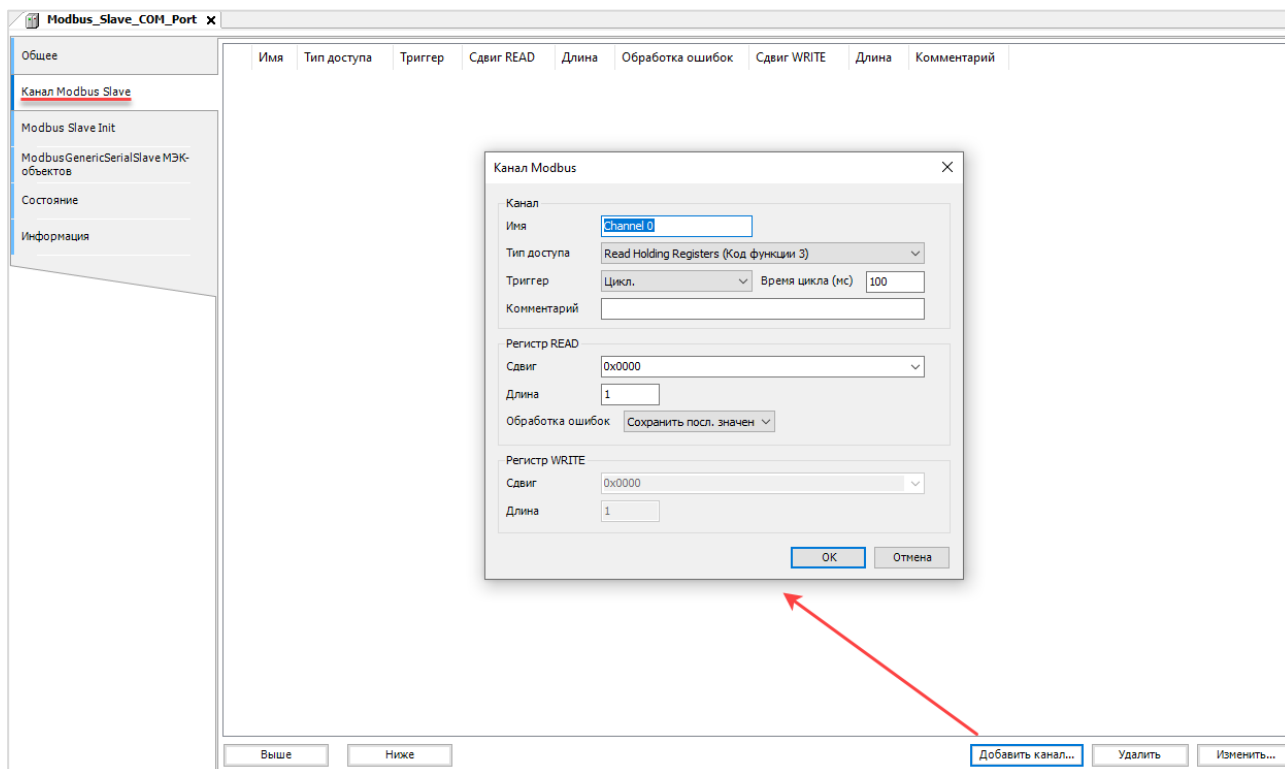
Рисунок 4.2.7 – Добавление канала Modbus Slave
