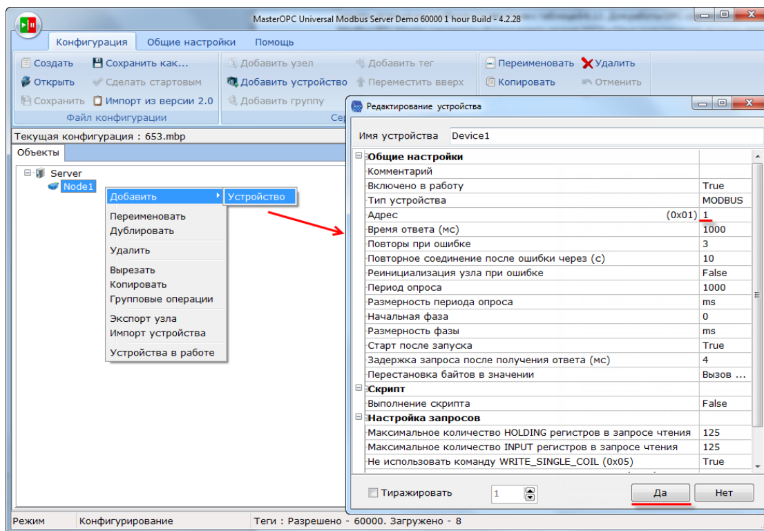
Рисунок 5.7.17 – Добавление устройства
