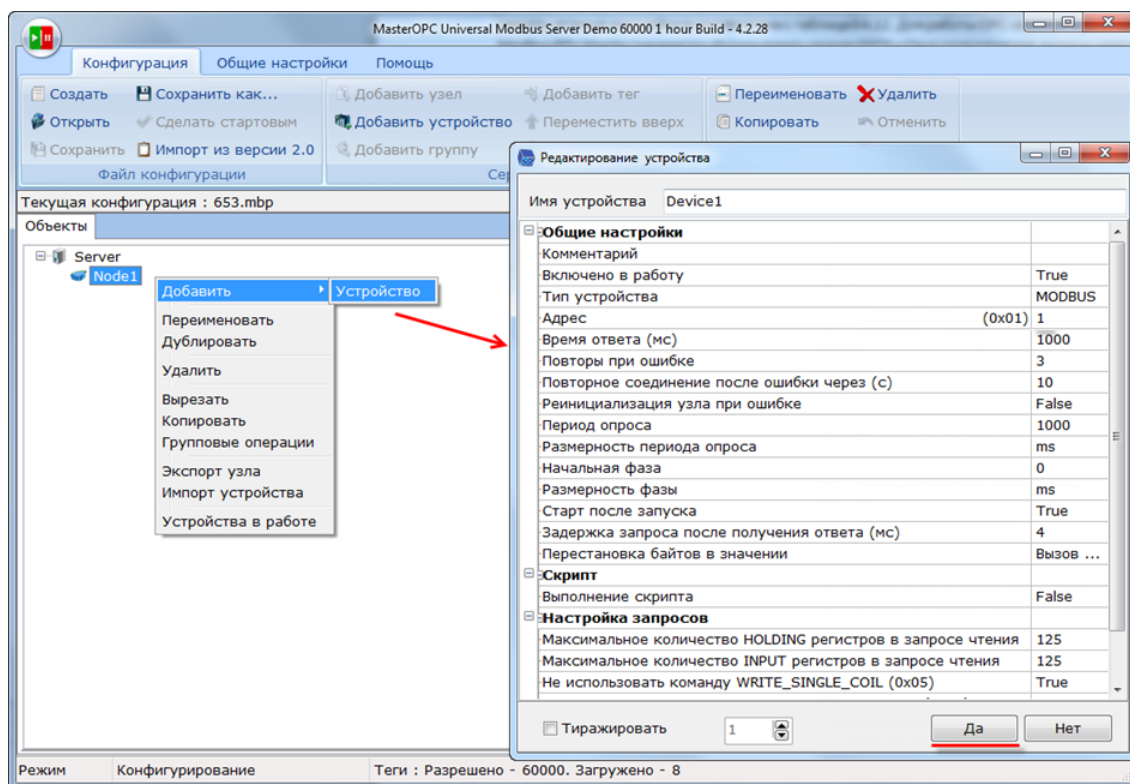
Рисунок 4.12.11 – Добавление устройства
