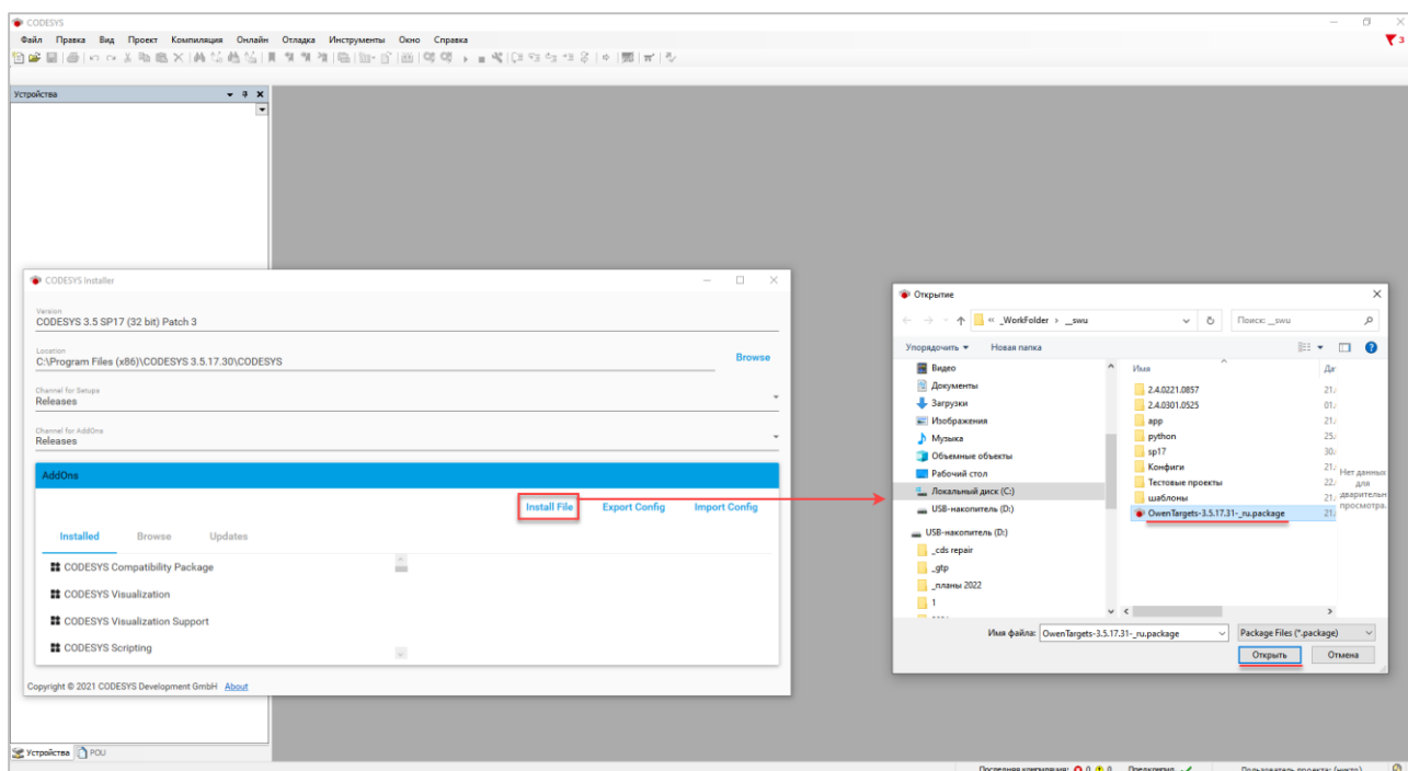
Рисунок 5.2 – Выбор пакета
