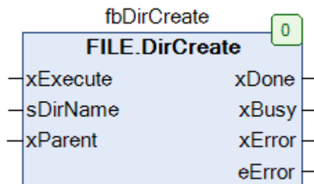
Рисунок 4.5.1 – Внешний вид ФБ FILE.DirCreate на языке CFC
