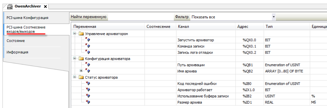
Рисунок 3.2.4 – Настройки архиватора, вкладка PCI-шина Соотнесение входов/выходов
