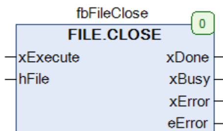
Рисунок 4.10 – Внешний вид ФБ FILE.Close на языке CFC
