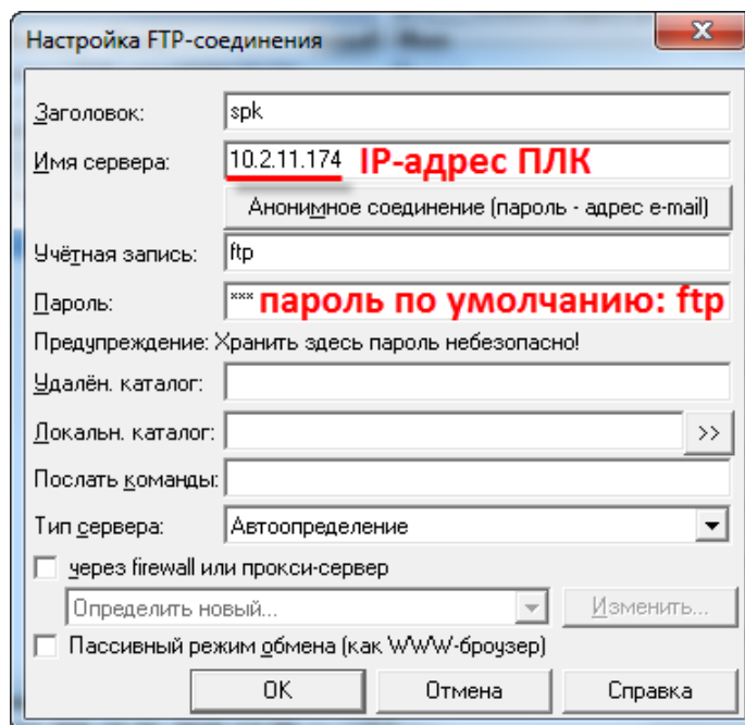
Рисунок 9.7 – Настройки FTP-соединения в файловом менеджере Total Commander
