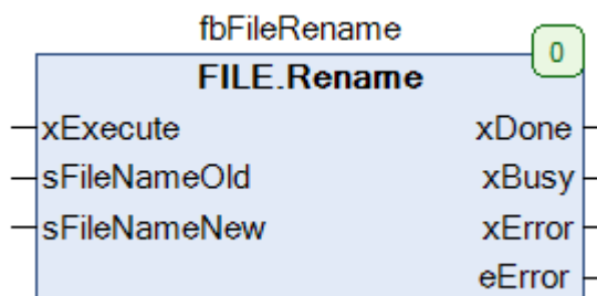
Рисунок 4.13 – Внешний вид ФБ FILE.RENAME на языке CFC
