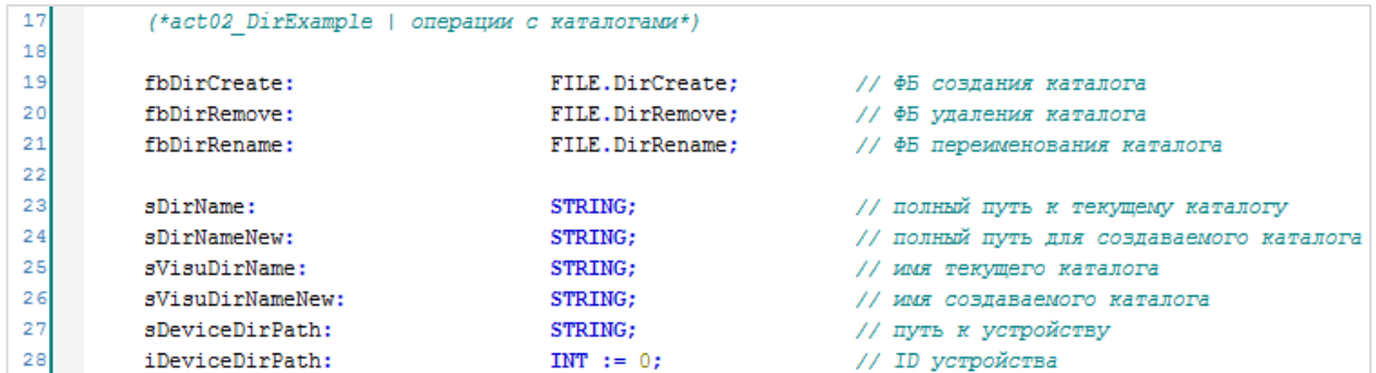
Рисунок 5.5.2 – Объявление переменных в программе PLC_PRG
