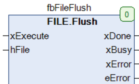
Рисунок 4.16 – Внешний вид ФБ FILE.FLUSH на языке CFC
