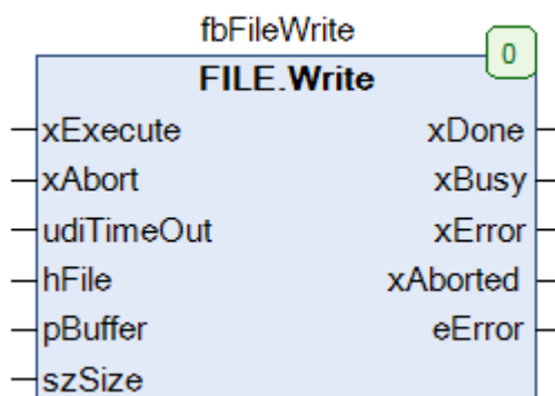
Рисунок 4.11 – Внешний вид ФБ FILE.WRITE на языке CFC
