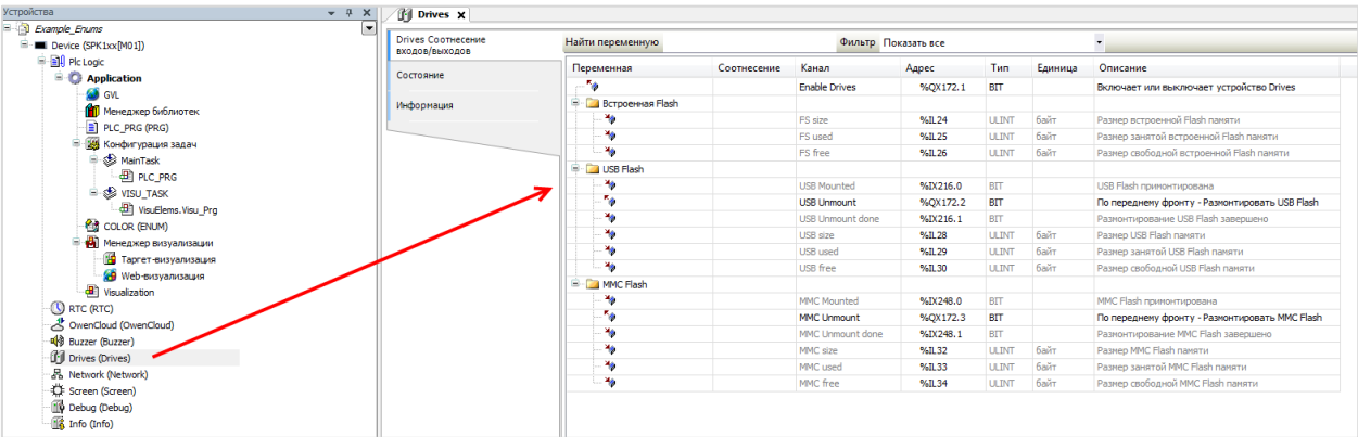
Рисунок 2.3 – Каналы узла Drives
