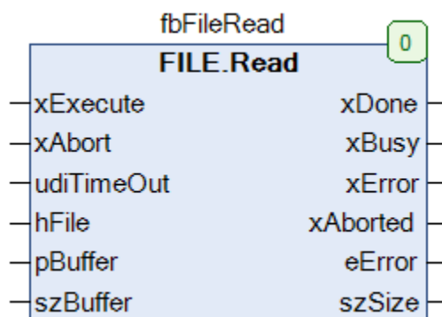
Рисунок 4.12 – Внешний вид ФБ FILE.READ на языке CFC
