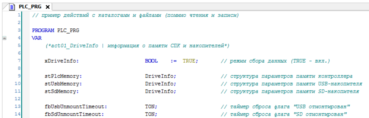
Рисунок 5.4.3 – Объявление переменных в программе PLC_PRG
