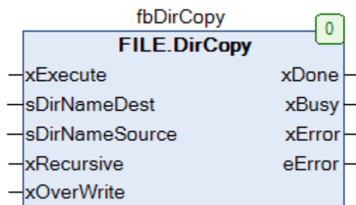
Рисунок 4.8 – Внешний вид ФБ FILE.DirCopy на языке CFC
