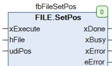
Рисунок 4.18 – Внешний вид ФБ FILE.SetPos на языке CFC
