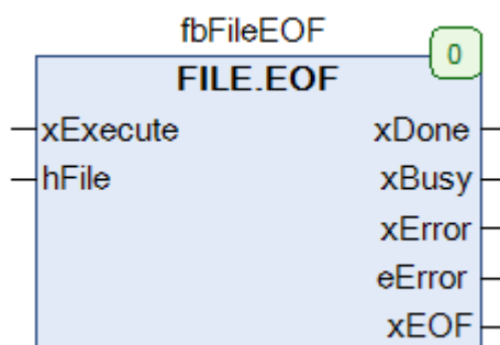
Рисунок 4.19 – Внешний вид ФБ FILE.EOF на языке CFC
