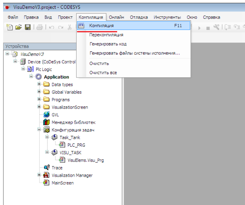
Рис. 7.26. Компиляция проекта
