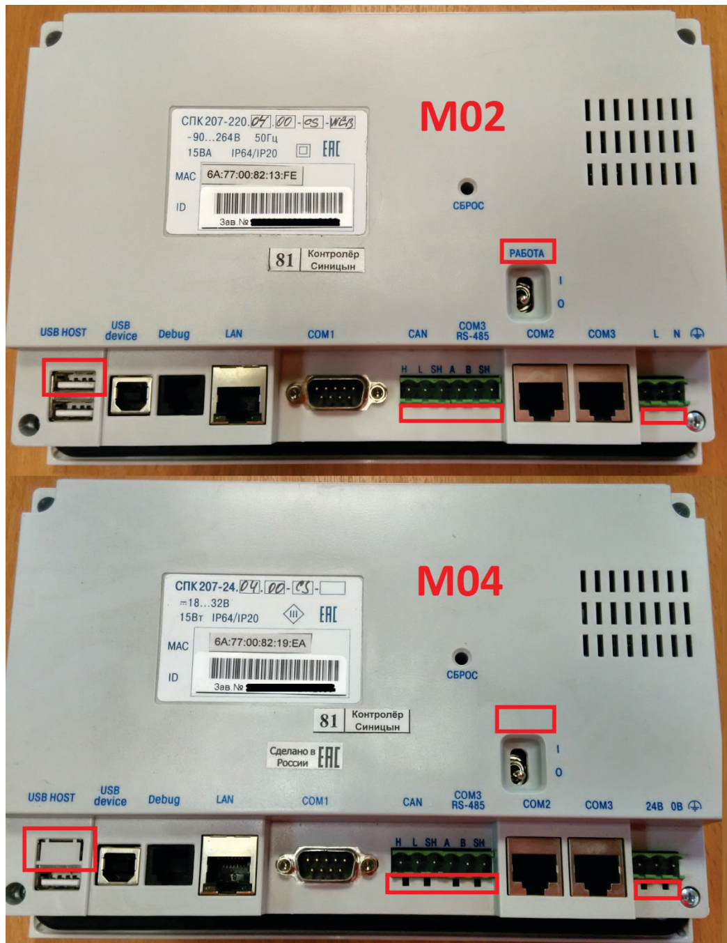
Рис. 6.3. Визуальные отличия M02 и M04
