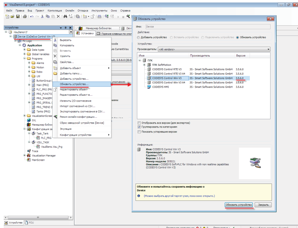
Рис. 7.37. Обновление target-файла
