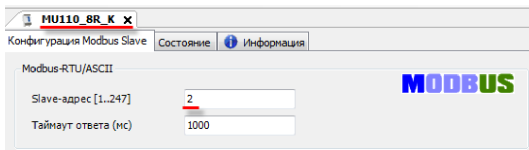
Рис. 7.150. Настройки модуля MU110_8R_K
