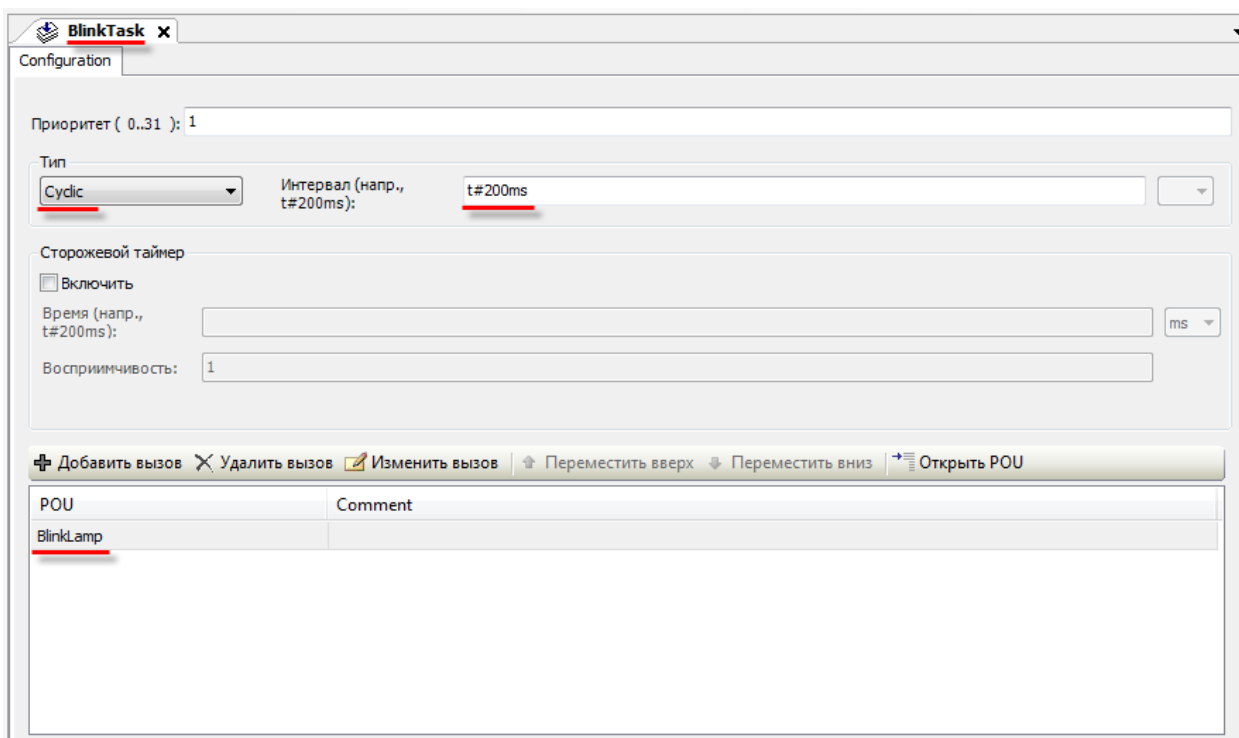
Рис. 7.140. Настройки задачи BlinkTask
