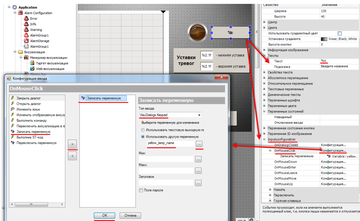
Рис. 7.121. Настройка поля ввода/отображения названия сигнальной лампы
