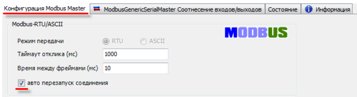
Рис. 7.147. Настройки компонента Modbus Master COM port
