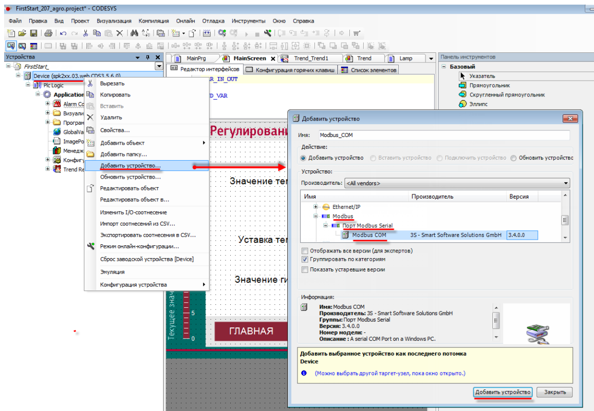
Рис. 7.144. Добавление компонента Modbus COM
