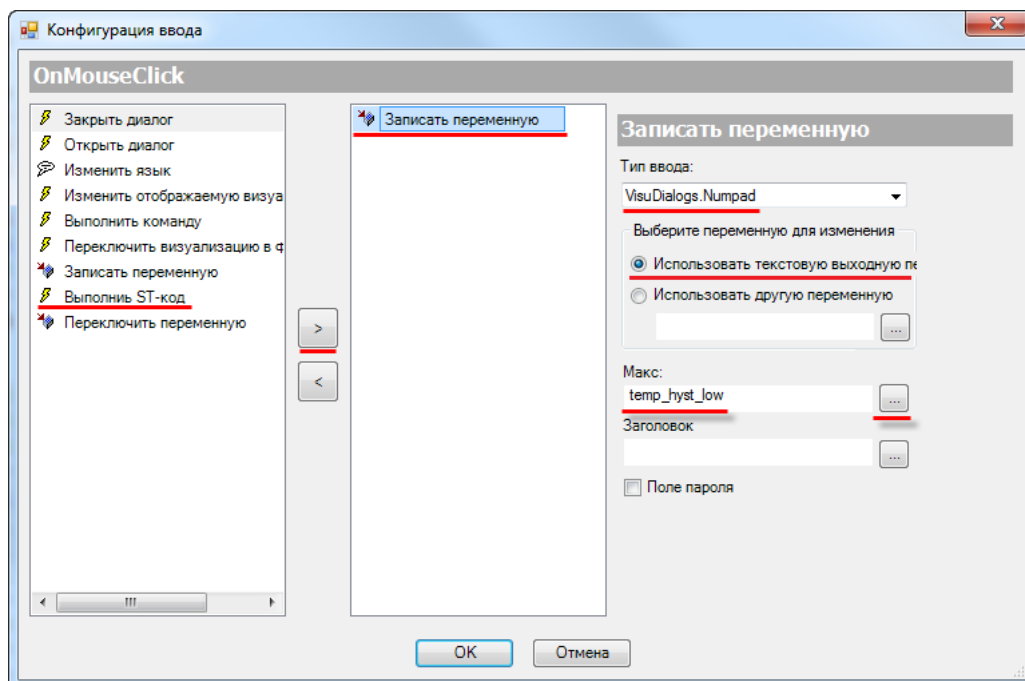
Рис. 7.122. Настройка действия поля нижней уставки тревоги
