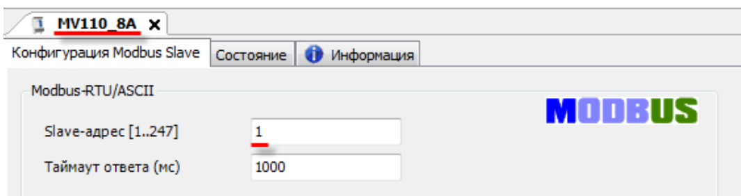
Рис. 7.149. Настройки модуля MV110_8A
